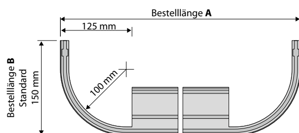
Retourenbiegung 4425/4430
