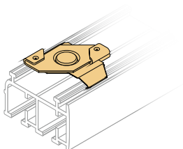
Schnellmontageclip mit Halteclip gekröpft für T-Profil 24–26 mm, nur geeignet für Schiene 7620 und 7630
