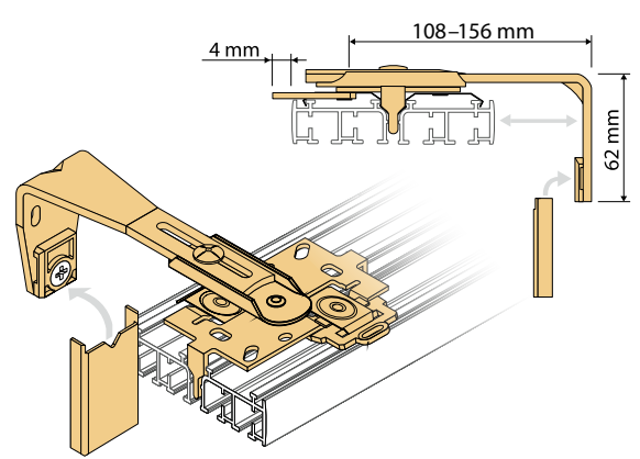
Wandwinkel 108-156 inklusive Abdeckkappe groß für 4- / 5-Lauf für 6-Lauf
