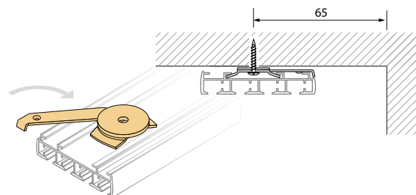
Deckenspanner für 4- / 5-Lauf-Schiene min. Wandabstand 65 mm
