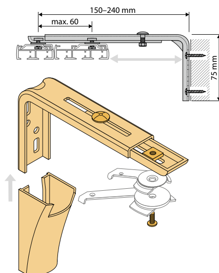
Wandwinkel inklusive Abdeckkappe Verstellbereich 150–240 mm
