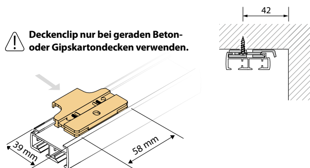
Deckenclip für Schiene 7520 und 7530
