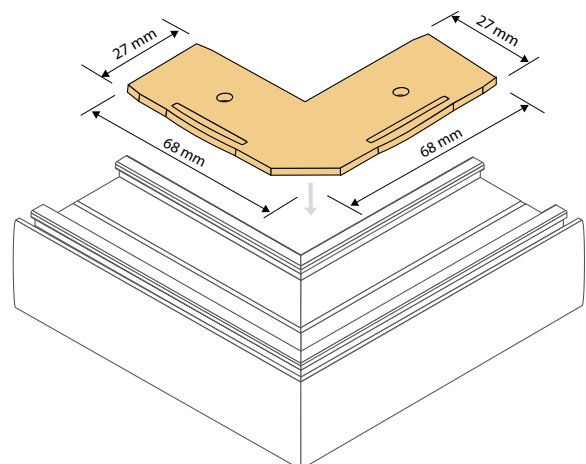
Eckverbinder
