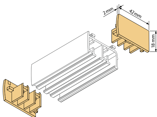
Endkappenpaar 2-Lauf
