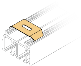
Halteclip gekröpft mit Langloch für 2- / 3- Lauf Schiene
