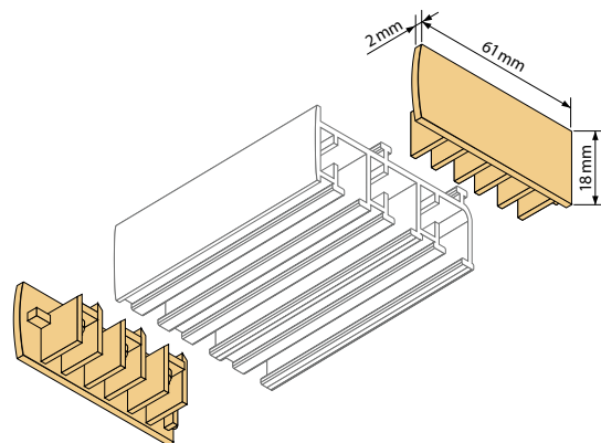
Endkappenpaar 3-Lauf
