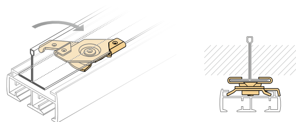
Schnellmontageclip mit Deckenspanner
