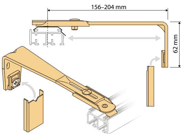
Wandwinkel 156-204 inklusive Abdeckkappe groß für 2- / 3-Lauf
