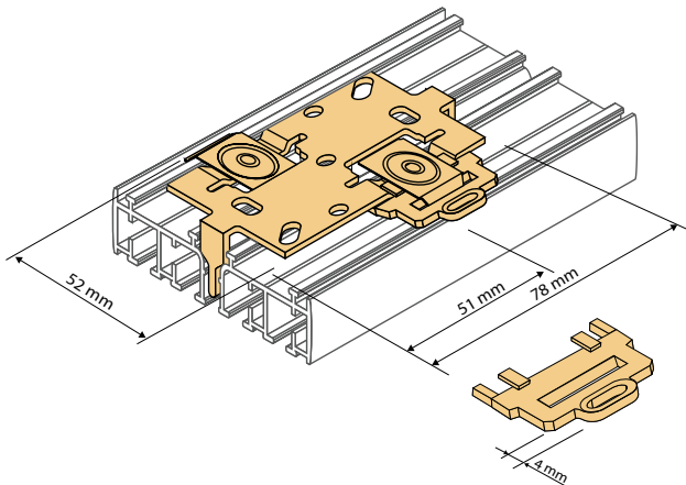
Deckendoppelhalter für 4- / 5-Lauf inkl. Auslöseplatte, Aufbauhöhe 4 mm
