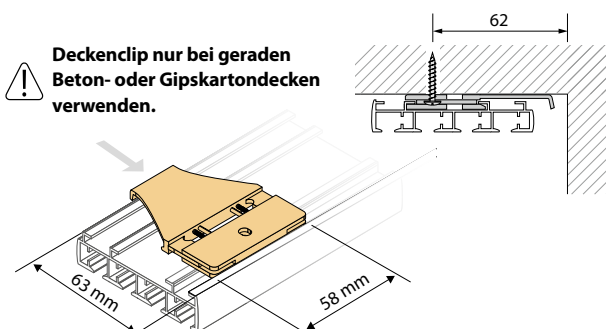
Deckenclip für Schiene 7540 und 7550
