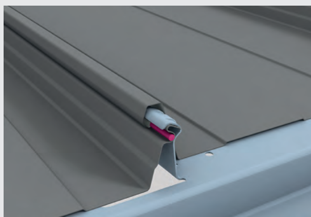
Profilübergreif Längsstoßdichtung mit Halteprofil
