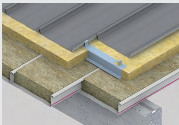
Zweischaliger wärmegeädmmter nichtbelüfteter Dachaufbau auf Betonpfetten mit Kassetten-Unterschale – Halteprofil „Z“
