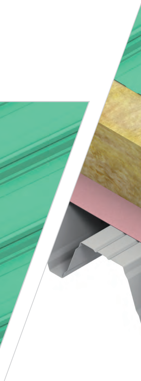
GBS Litkuppel-Anschluss firstseitig – Kassetten-Unterschale auf Stahlbinder
