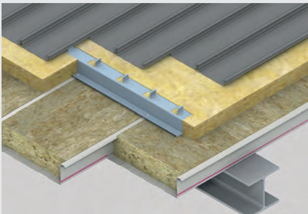
Zweischaliger wärmegeädmmter nichtbelüfte- ter Dachaufbau auf Stahlpfetten mit Kassetten- Unterschale – Halteprofil „Z“
