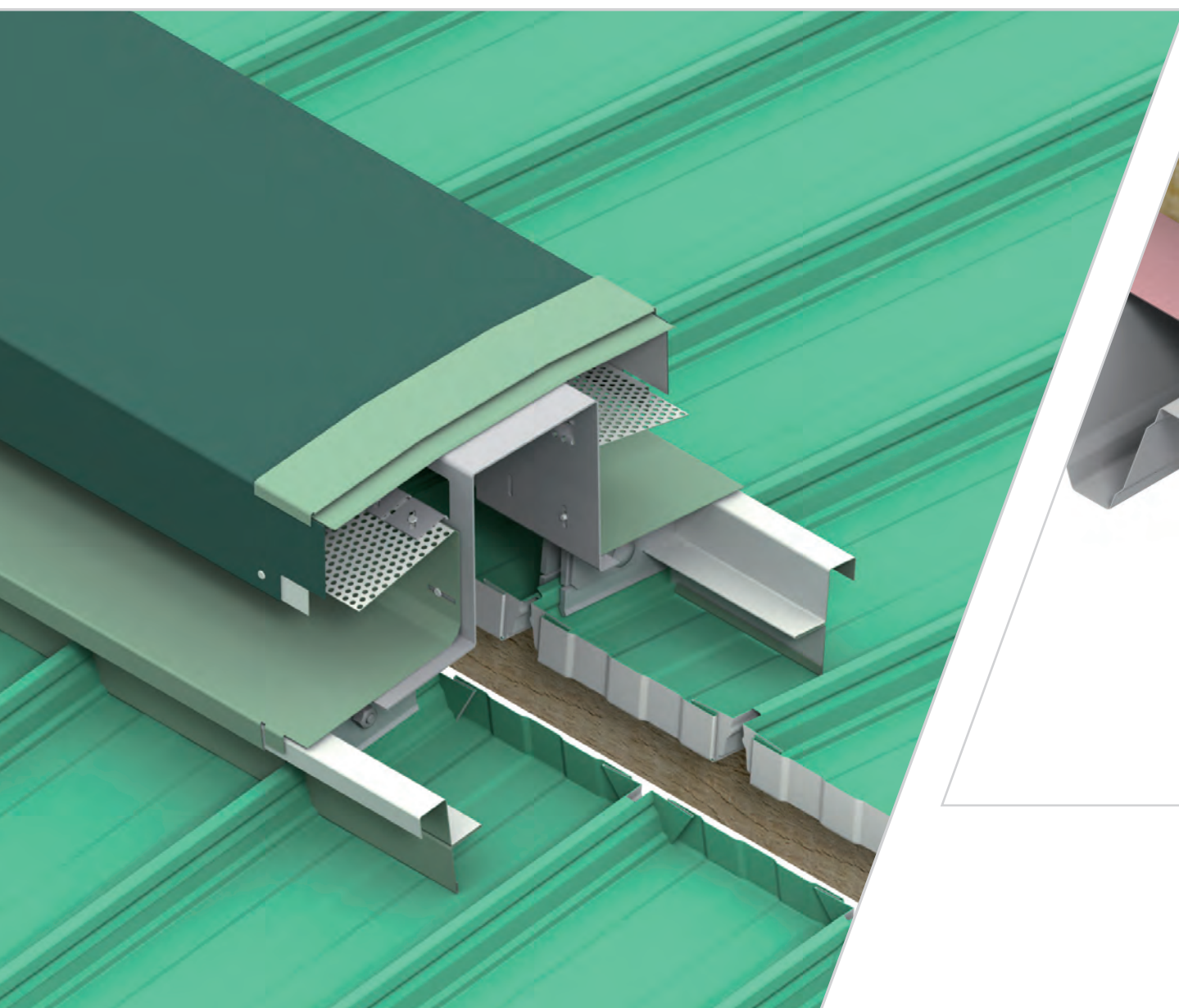
GBS Lüfterfirst-Ausbildung auf Holzpfetten
