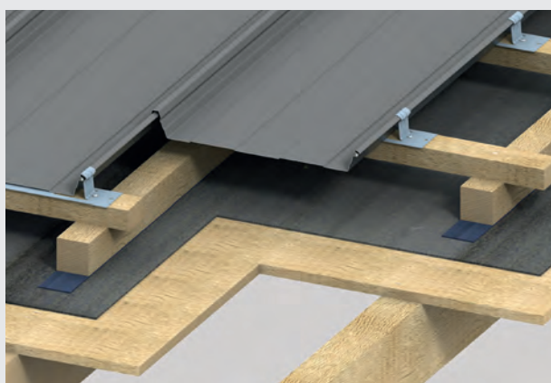
Einschaliger ungedämmter belüfteter Dachaufbau auf Holzschalung und Konterlattung mit Halteprofil „L“
