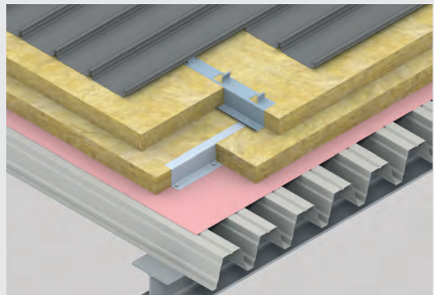
Zweischaliger wärmegeädmmter nichtbelüfte- ter Dachaufbau auf Stahlbinder mit Trapezprofil- Unterschale – Halteprofil „Z“
