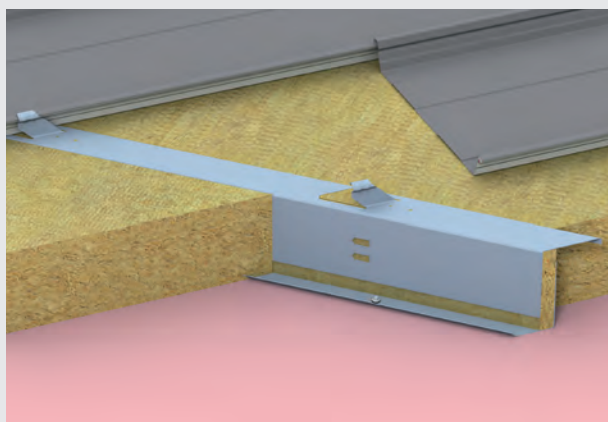
Zweischaliges wärmegeädmmtes nichtbelüftetes Dach mit Trapezprofil-Unterschale auf Binder – Halteprofil „S“ 45° mit thermischer Trennung
