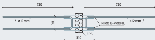
Abb. 2: Rippenausführungen der Typenreihe SL-TKM
