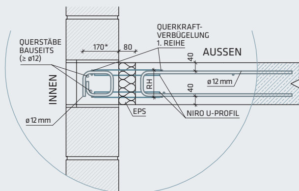
Abb. 8: Loggia mit SL-TKA/C G-Q1-Rippe
