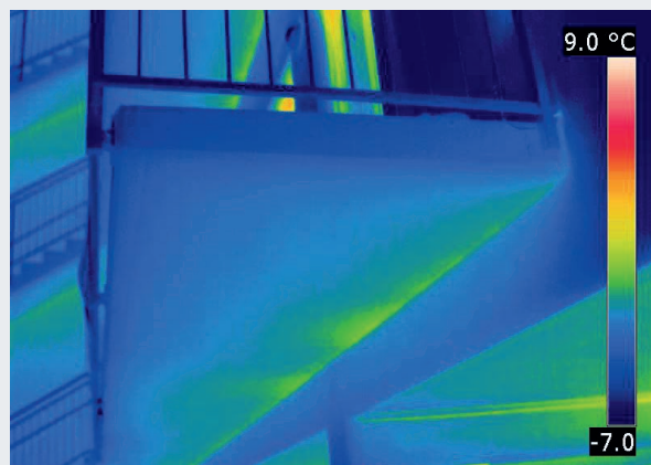
Abb. 15: Anschlussbereich mit Thermokorb® TK
