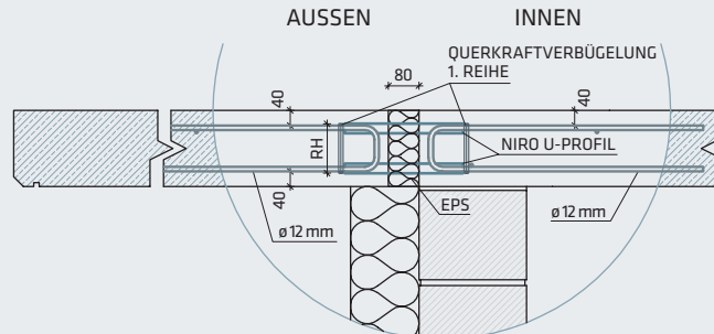
Abb. 3: Ausragende Balkonplatte mit SL-TKM/C G-G-Rippe
