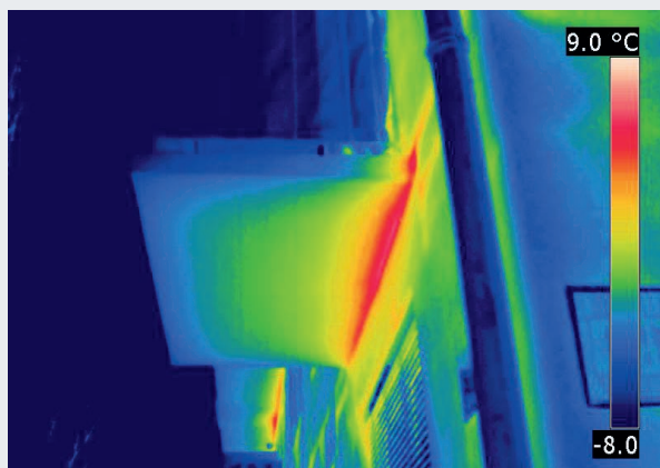
Abb. 14: Ungedämmter Anschlussbereich
