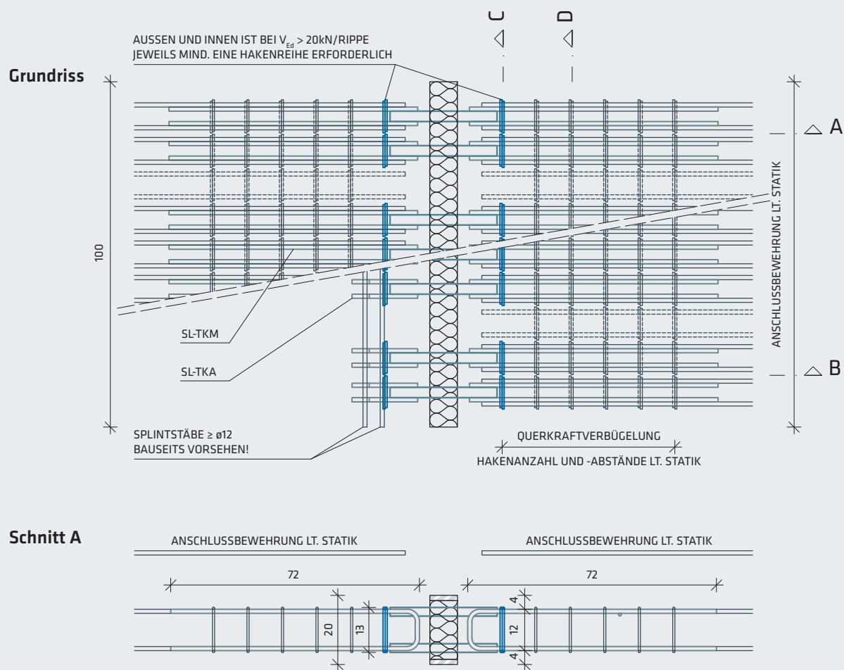
Abb. 10: Bauseitige Bewehrung SL-TKM und SL-TKA (Grundriss und Schnitt A)
