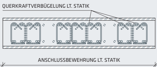
Abb. 11: Bauseitige Bewehrung SL-TKM und SL-TKA (Schnitt B, Schnitt C und Schnitt D)
