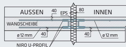
Abb. 9: Wandanschluss mit SL-TKM/C G-G-Rippe (Grundriss, Ansicht und Schnitt)
