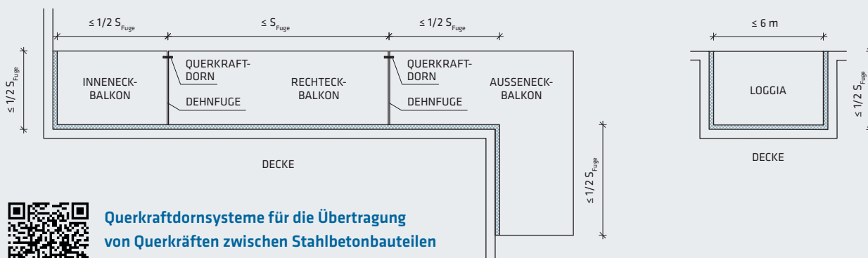
Abb. 12: Dehnfugenabstände
