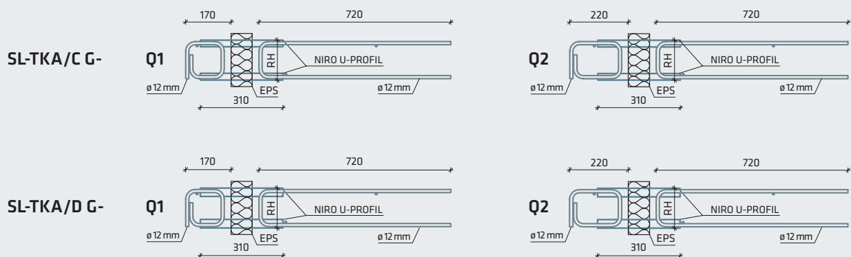
Abb. 6: Rippenausführungen der Typenreihe SL-TKA
