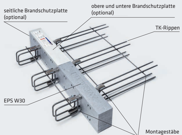
Abb. 5: SL-TKA/C G-Q2 beispielhaft mit/ohne Brandschutzplatten
