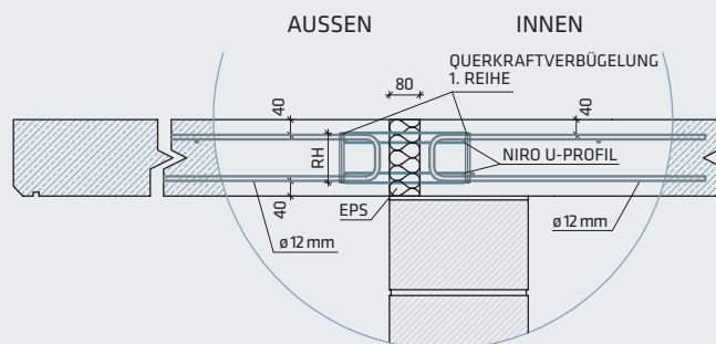
Abb. 4: Ausragende Balkonplatte mit SL-TKM/C G-G-Rippe
