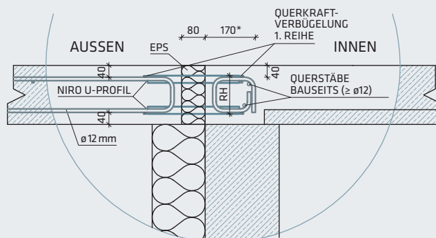
Abb. 7: Gestützter Balkon mit SL-TKA/C G-Q1-Rippe
