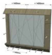
Bild 8: Sicherungsschrauben BLK-Tür 3-flg.
