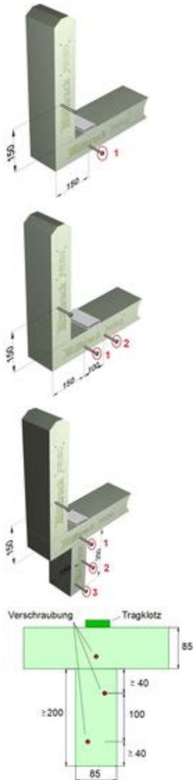
Stützklötz
