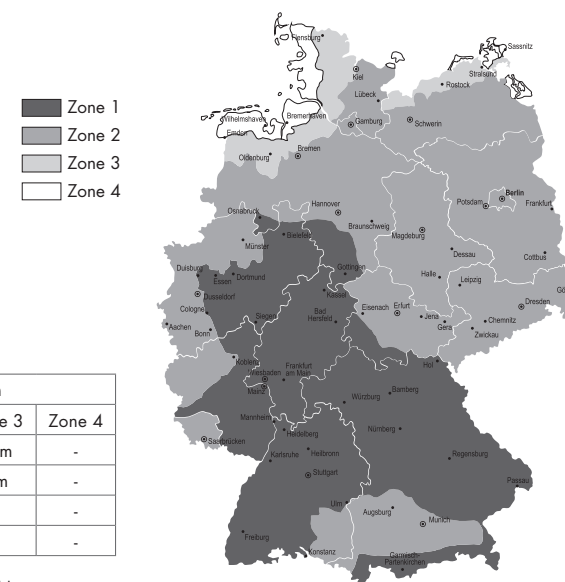
Deutschland – Windzonen gemäß EN 1991-1-4 (1995)
