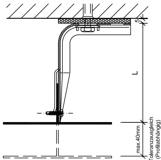
TOLERANZAUSGLEICH
