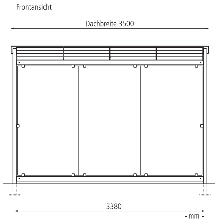
Fahrradüberdachung PICTOR, Dachbreite x Dachtiefe 3500 mm x 2250 mm, mit Rück- / Seitenwände aus ESG Klarglas, mit Anlehnbügel FLORIDA, Stahlkonstruktion in RAL 7016 anthrazitgrau
