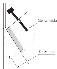
▲ Einwurföffnung einstellbar
