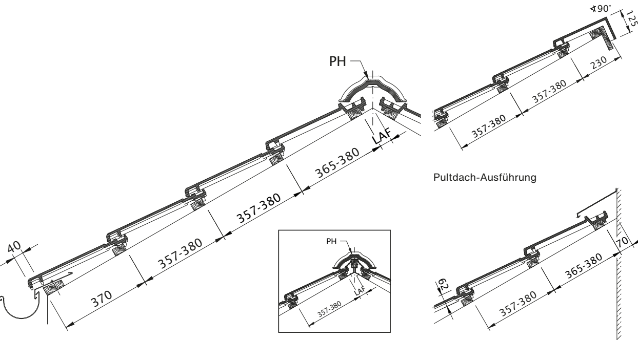
Dachquerschnitt Entlüftung über FALZ. Firstziegel trocken verlegt. LQ bis ca. 230 cm 2 /lfm First. Wandanschluss (oben) mit Firstanschluss- Lüfterziegel
