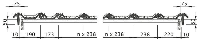
Ortgangausbildung mit Ortgangziegel links mit Ortgangbrett Ortgangausbildung mit Ortgangziegel rechts mit Ortgangbrett Der Abstand bei Ortgangziegeln soll zwischen Innenkante Ortganglappen und Außenkante Bekleidung mindestens 1 cm betragen. Die dargestellten Zeichnungen sind nur Konstruktionsbeispiele. Bei der Ausführung sind die nationalen Regelwerke zu beachten.
