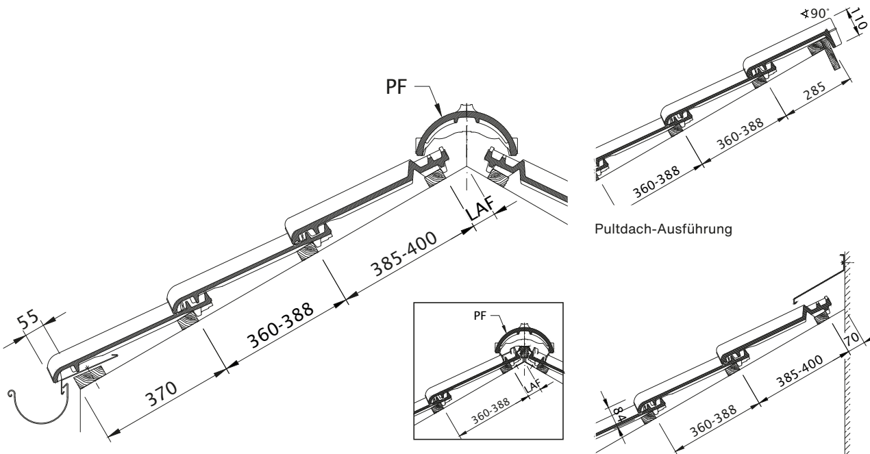
Dachquerschnitt Entlüftung über FALZ. Firstziegel trocken verlegt. LQ bis ca. 230 cm 2 /lfm First. Traufplattenabstand variabel. Wandanschluss (oben) mit Firstanschluss- Lüfterziegel
