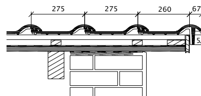
Ortgangausbildung mit Ortgangziegel rechts mit Ortgangbrett
