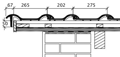
Ortgangausbildung mit Ortgangziegel links mit Ortgangbrett
