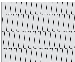
Einfachdeckung Steinschindel 38,5x19,4 cm
