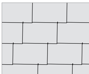
Einfachdeckung Rechteck 40x60 cm
