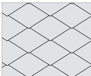
Einfachdeckung Rhombus Schablone 40x44 cm
