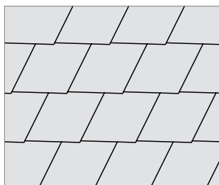
Einfachdeckung Rhombus 40x44 cm
