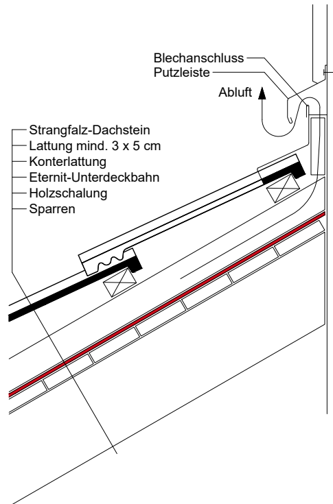
Wandanschluss - Firstseitig
