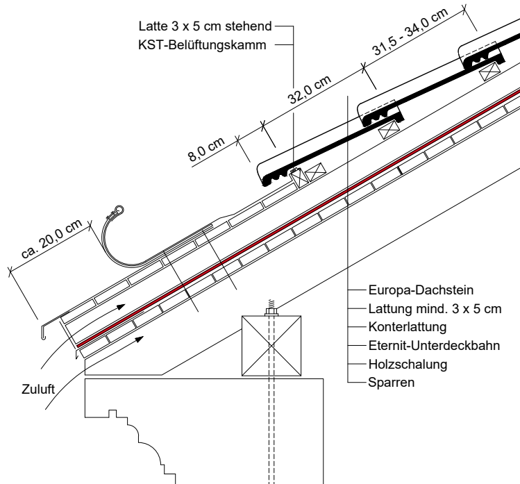
Traufe mit Saumrinne
