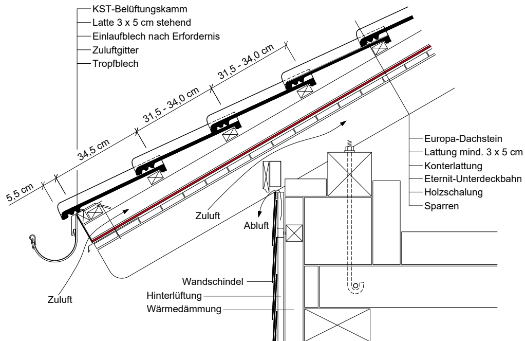
Europa-Dachstein
