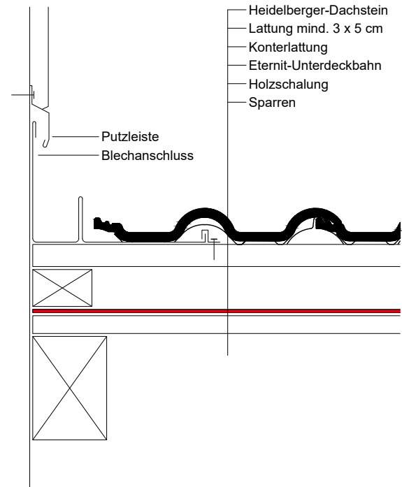
Wandanschluss - seitlich
