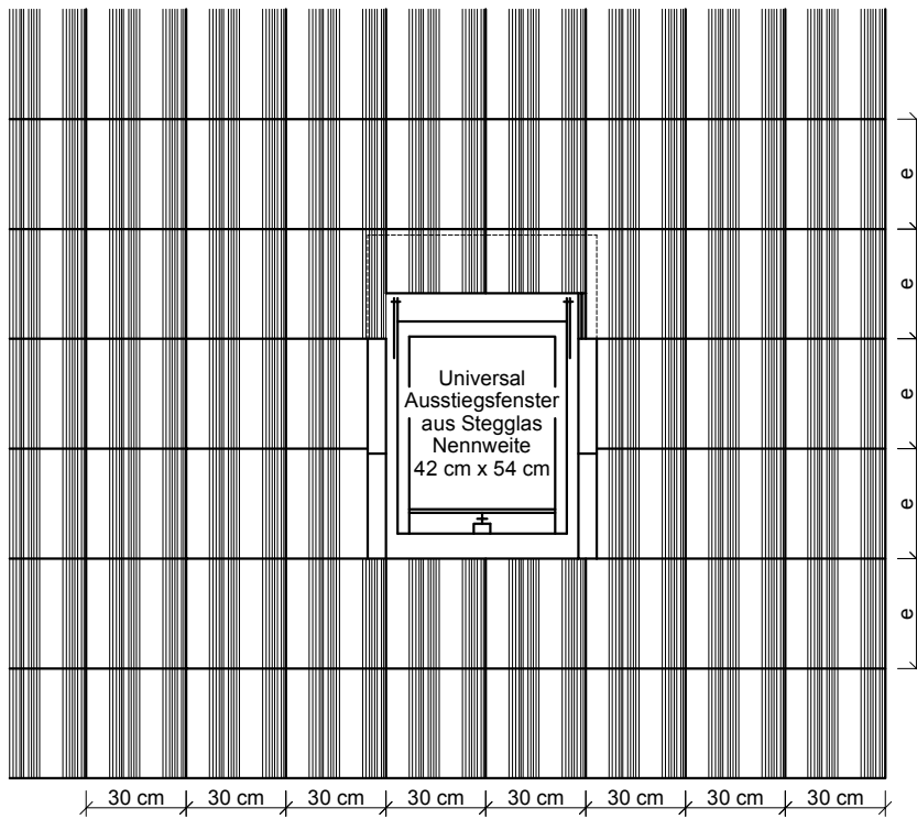
Ausstiegsfenster aus Stegglas
