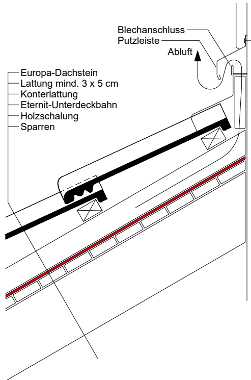
Wandanschluss - Firstseitig
