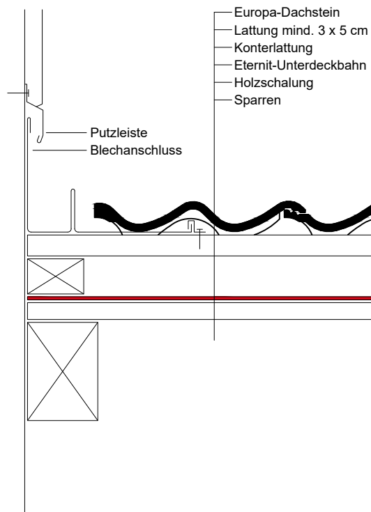
Wandanschluss - seitlich
