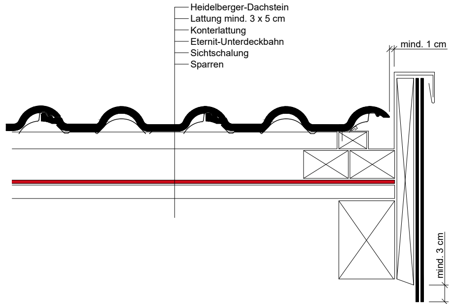
Heidelberger-Dachstein
