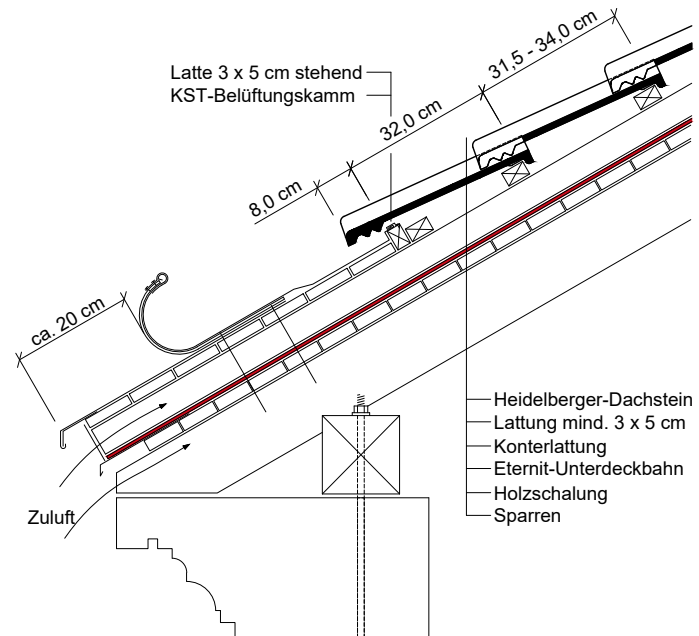
Traufe mit Saumrinne
