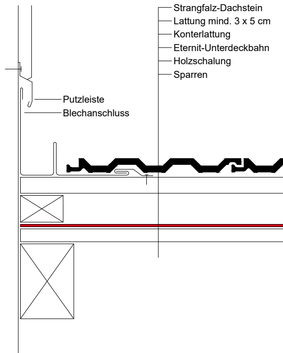
Wandanschluss - seitlich
