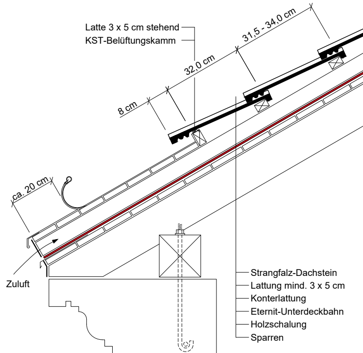
Traufe mit Saumrinne und Unterdach
