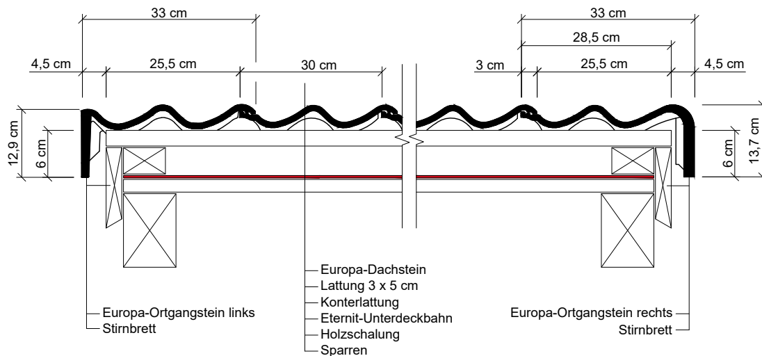
Europa-Dachstein
