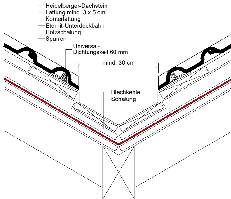
Kehle in Blech
