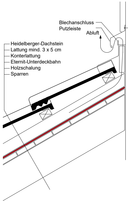
Wandanschluss - Firstseitig
