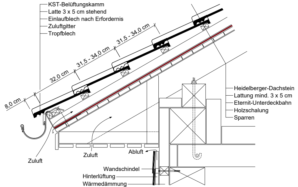
Traufe
