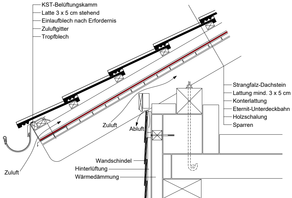
Strangfalz-Dachstein
