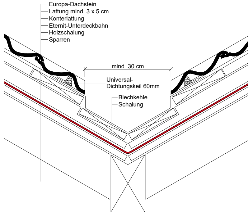
Kehle in Blech
