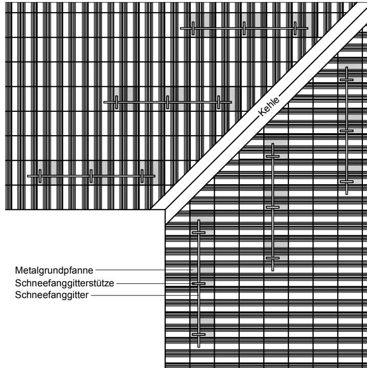
Kehle bei hohen Schneelasten
