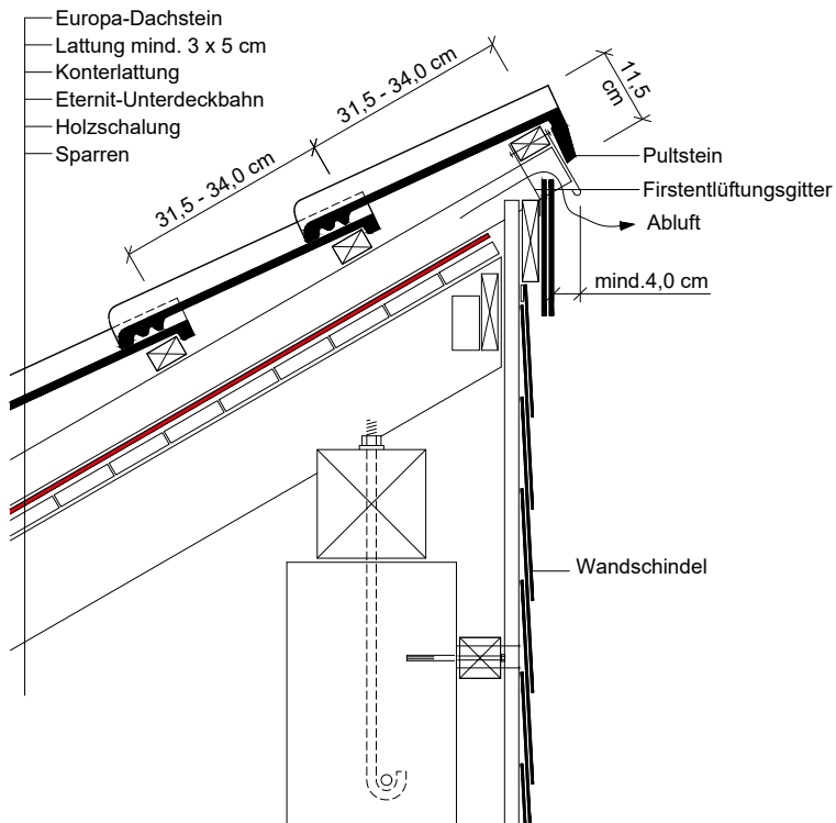
Halbfirst mit Europa-Pultstein
