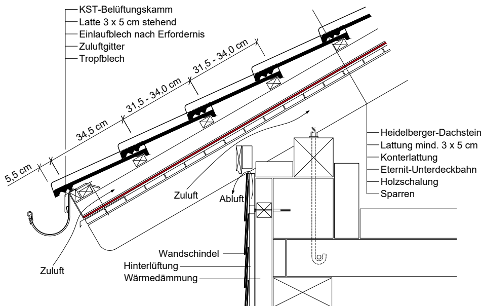
Traufe bei hohen Schneelasten
