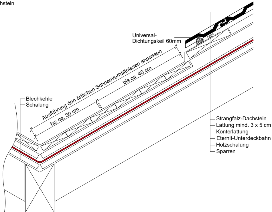
Kehle in Blech bei erhöhten Schneelasten
