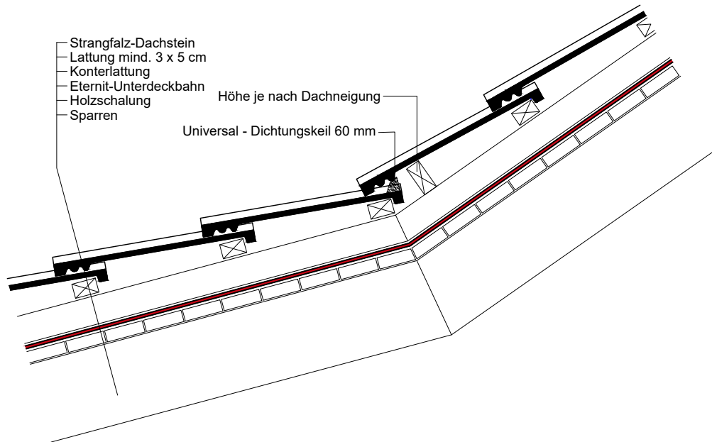
Strangfalz-Dachstein
