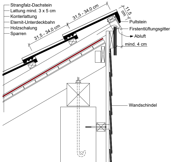
Halbfirst mit Strangfalz-Pultstein
