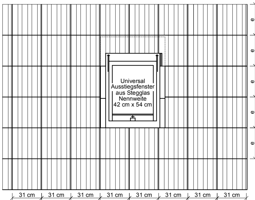
Ausstiegswindow aus Stegglas
