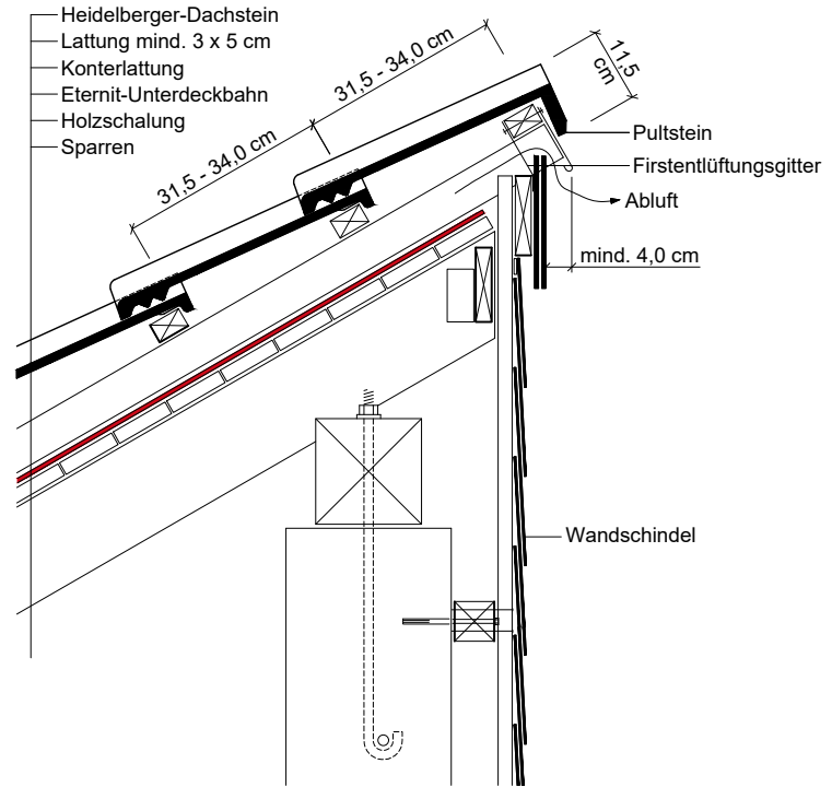
Halbfirst mit Heidelberger-Pultstein
