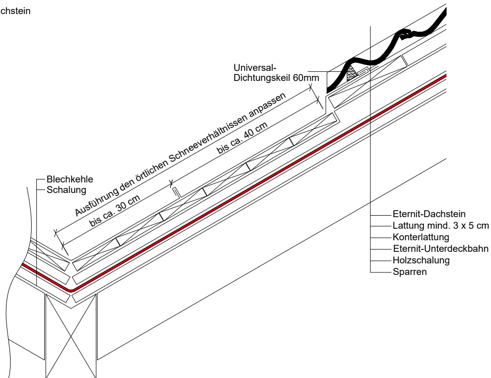
Kehle in Blech bei erhöhten Schneelasten
