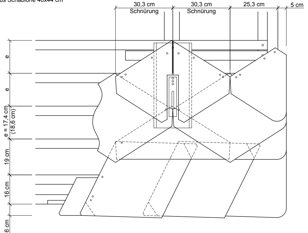
Traufe mit Rhombusstein - Ortgang mit Überstand
