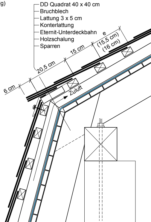
Dachnick bei Mansard-Dächer
