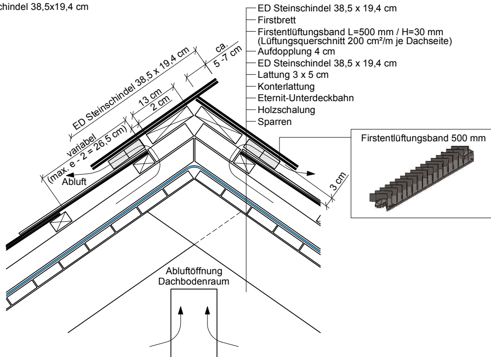
First mit wetterseitigen Überstand und Firstentlüftungsband (Entlüftungsquerschnitt 200 cm 2 /lfm First und Dachseite)
