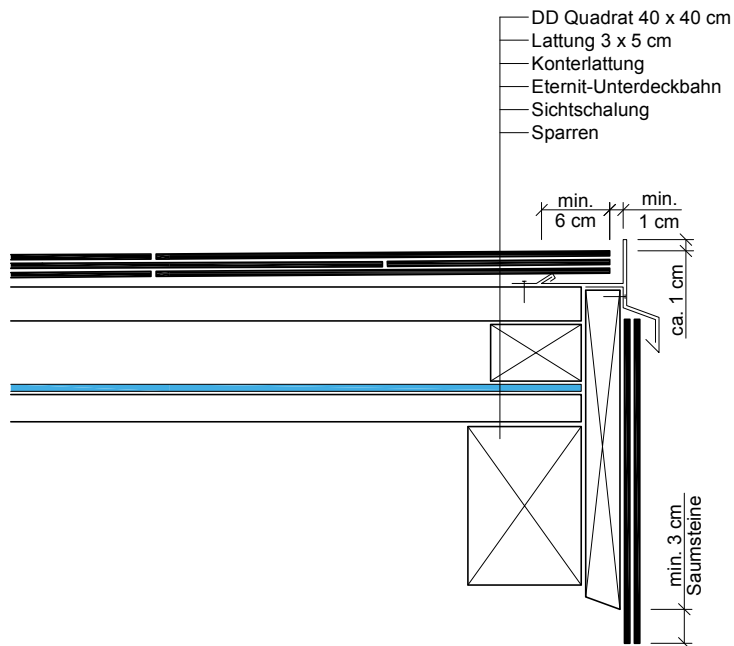
Ortgang mit Blech
