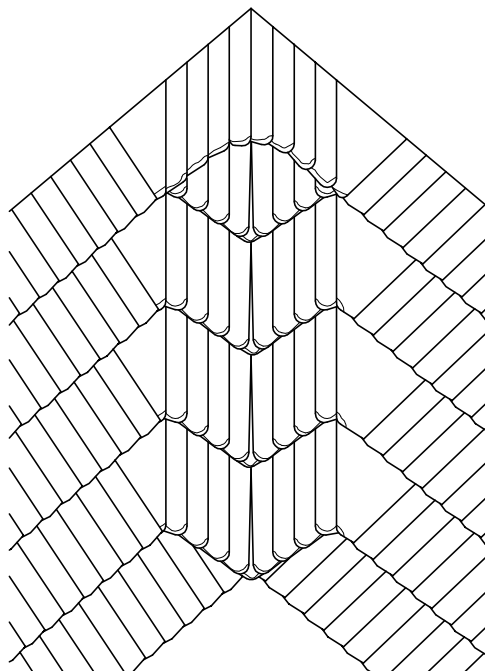
Herzkehle mit Kragengebäude als oberer Abschluss
