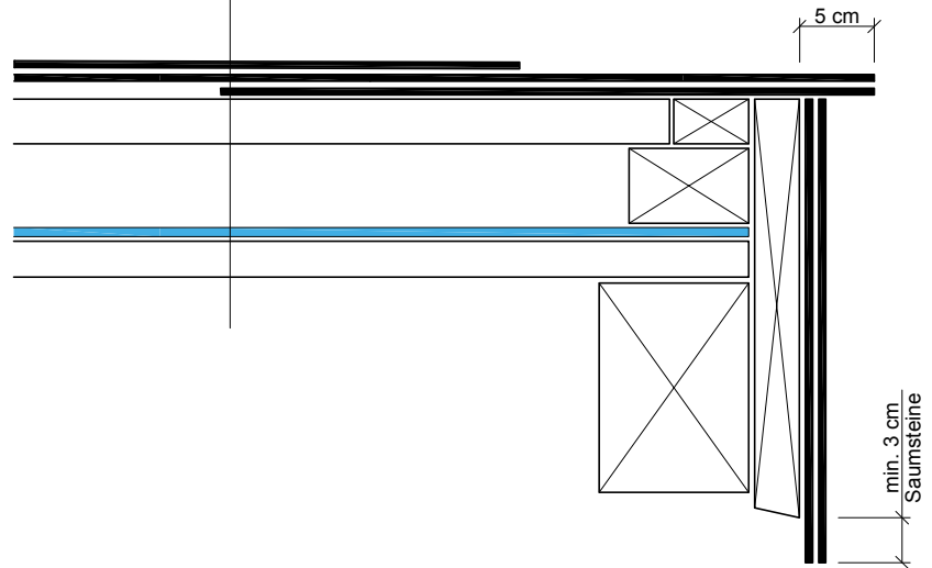
Ortgang mit Überstand
