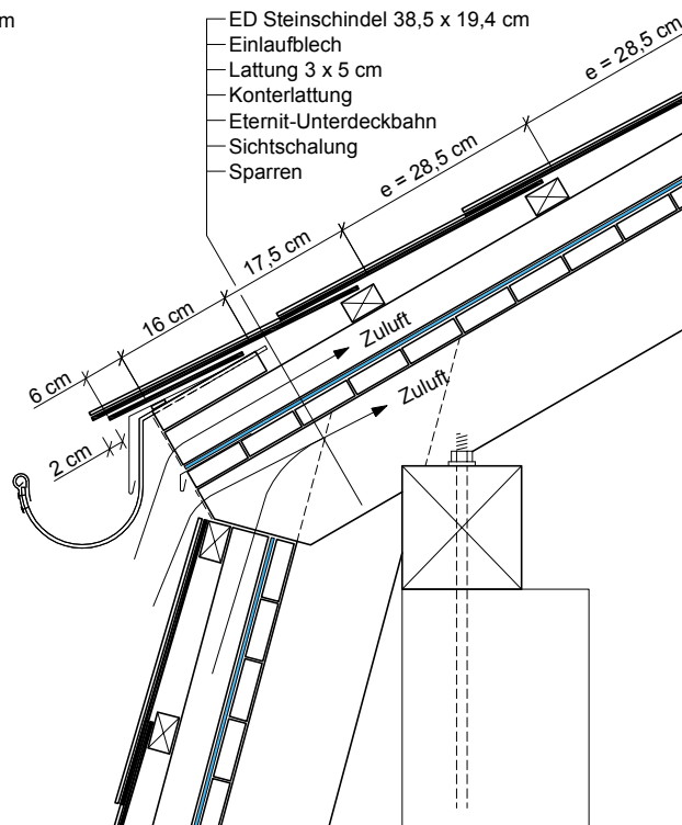
Dachknick mit Hängerinne
