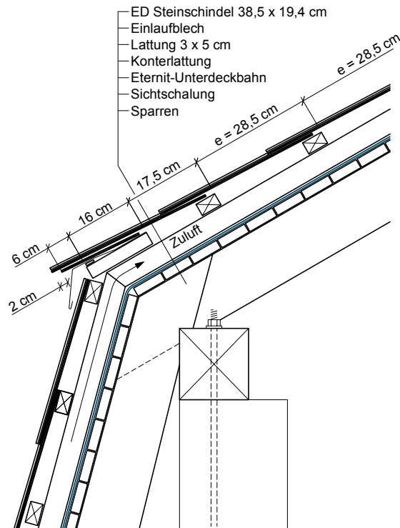
Dachknick bei Mansard-Dächern
