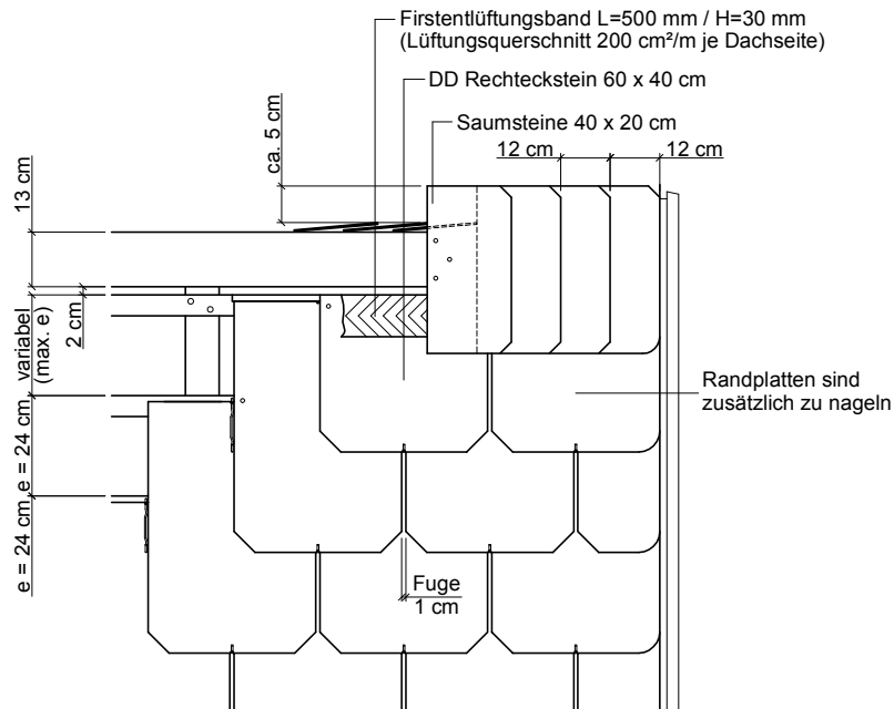
First mit Saumsteinen und Firstentlüftungsband (Entlüftungsquerschnitt 200 cm 2 /lfm First und Dachseite)
