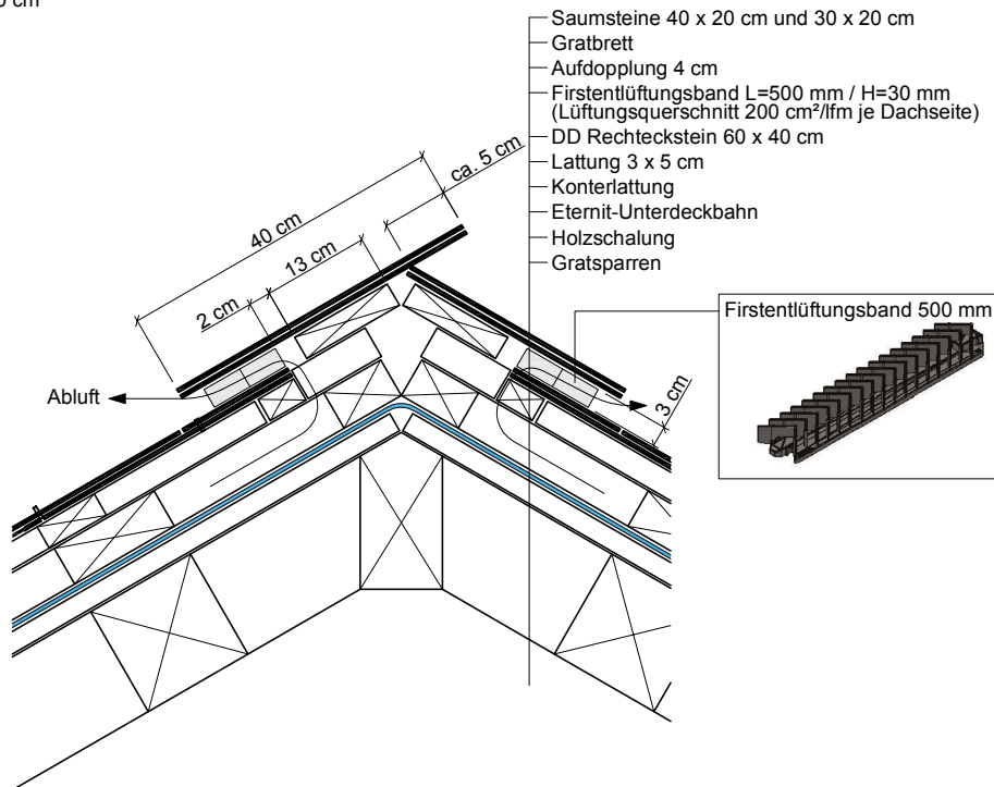
Grat mit Saumsteinen 30/20 & 40/20 cm (wetterseitiger Überstand) und Firstentlüftungsband (Entlüftungsquerschnitt 200 cm 2 /lfm First und Dachseite)
