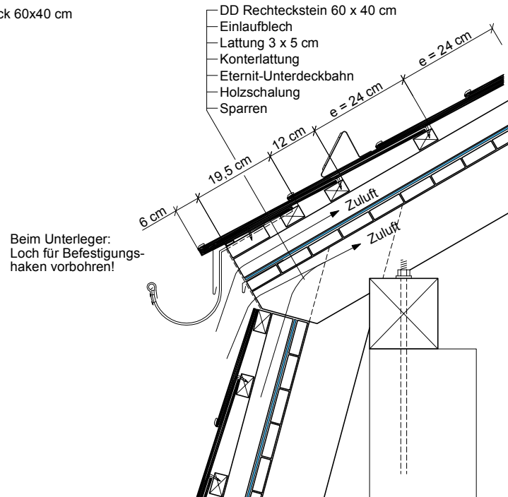
Dachknick mit Hängerinne
