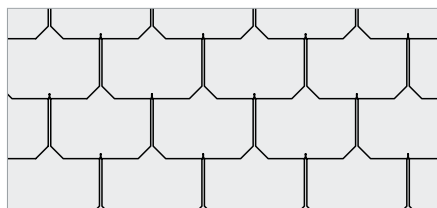
Doppeldeckung Rechteck 400 × 600 mm
