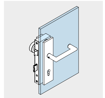
Uniquin Schloss mit Panikfunktion E (DIN 179) PZ-vorgerichtet, Panikfunktion D: C-Form Drücker auf Innenseite und feststehender Knopf auf Außenseite
