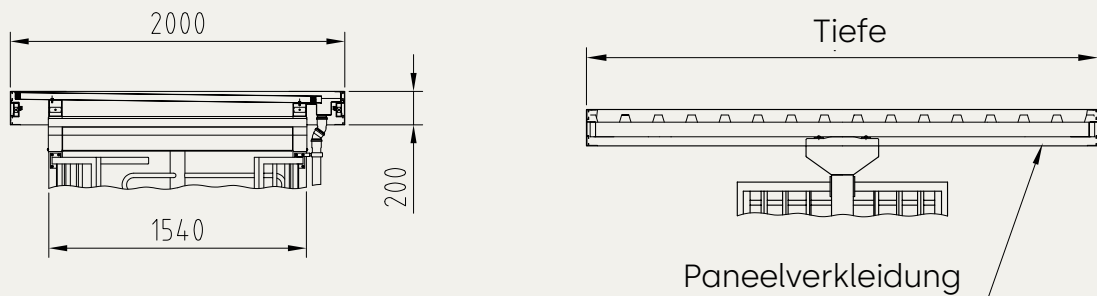
Dach D3 – mit Trapezblechabdeckung, Dachrandprofil, Paneelverkleidung und Wasserablauf
