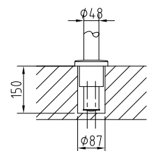
Spannelement
