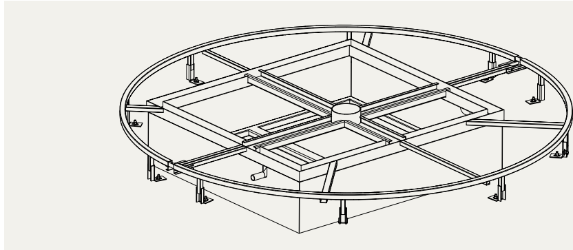
Bodenelement mit Antriebskasten für Bodengrube, ab Maß X = 350
