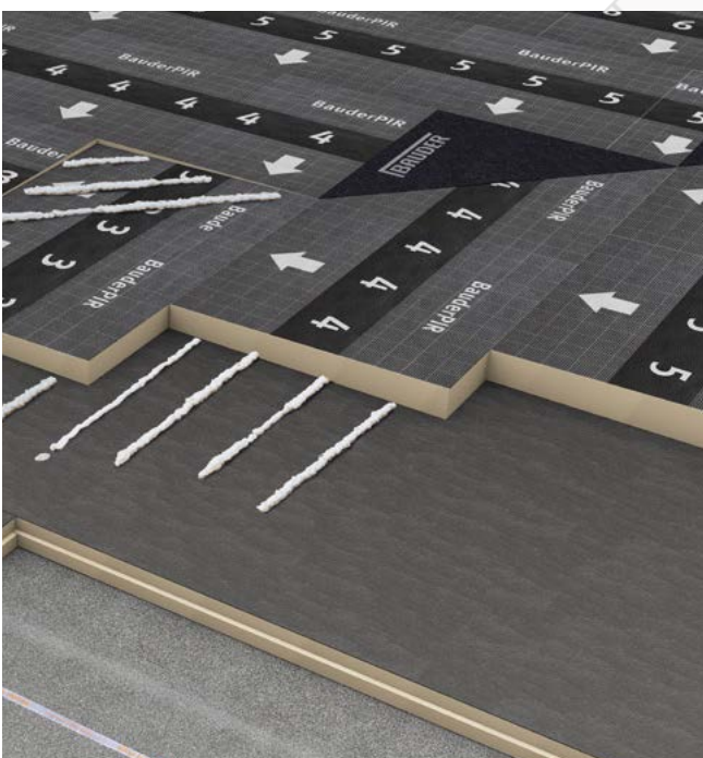
Abb. 6/1: Verlegebeispiel BauderPIR KFS G20 (Kehlfüllstück)
