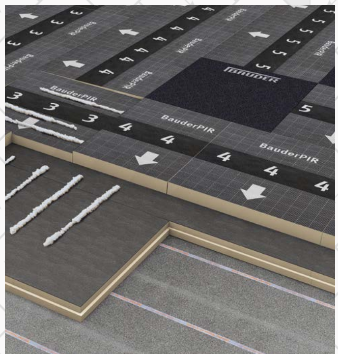
Abb. 6/2: Verlegebeispiel BauderPIR GFS G20 (Gratfüllstück)
