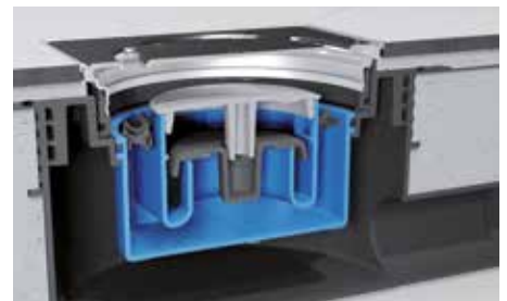
In trockenem Zustand, bedingt durch z. B. längere Nichtnutzung oder eine umgebende Fußbodenheizung, garantiert der mechanische Geruchsverschluss die dauerhafte Geruchsdichtheit
