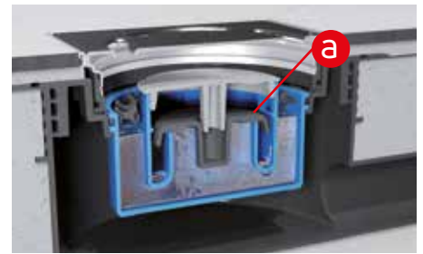
Wenn die Wasserzufuhr beendet wird, verschließt der Ventilteller (a) den Ventilsitz, das Sperrwasser verbleibt im Siphon
