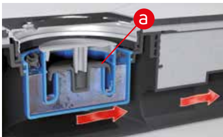
Bei kanalseitigem Unterdruck verhindert das Sperrwasser gemeinsam mit dem Gewicht des Ventiltellers (a) das Leersaugen des Siphons
