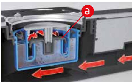
Bei kanalseitigem Überdruck wird der Ventilteller (a) gegen den Ventilsitz gedrückt und verhindert so das Austreten von Kanalgasen. Weiterer Vorteil: gegen Rückfluss gesichert
