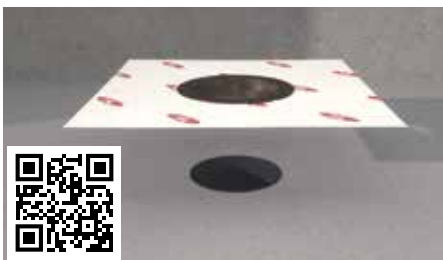
Abdichtgarnitur in den Ablauf einsetzen. Feuchtigkeitsabdichtung unter und ober der Abdichtgarnitur (Sandwichverfahren), sowie im gesamten Duschbereich auftragen. Alle Anschlussstellen mit bauseitigen Dichtbändern versehen.
