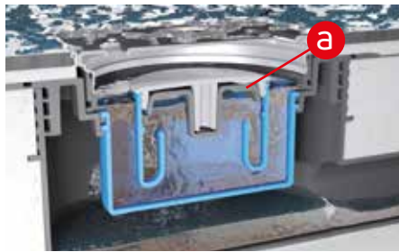
Bei geöffnetem Ventilteller (a) kann das Wasser ungehindert abfließen
