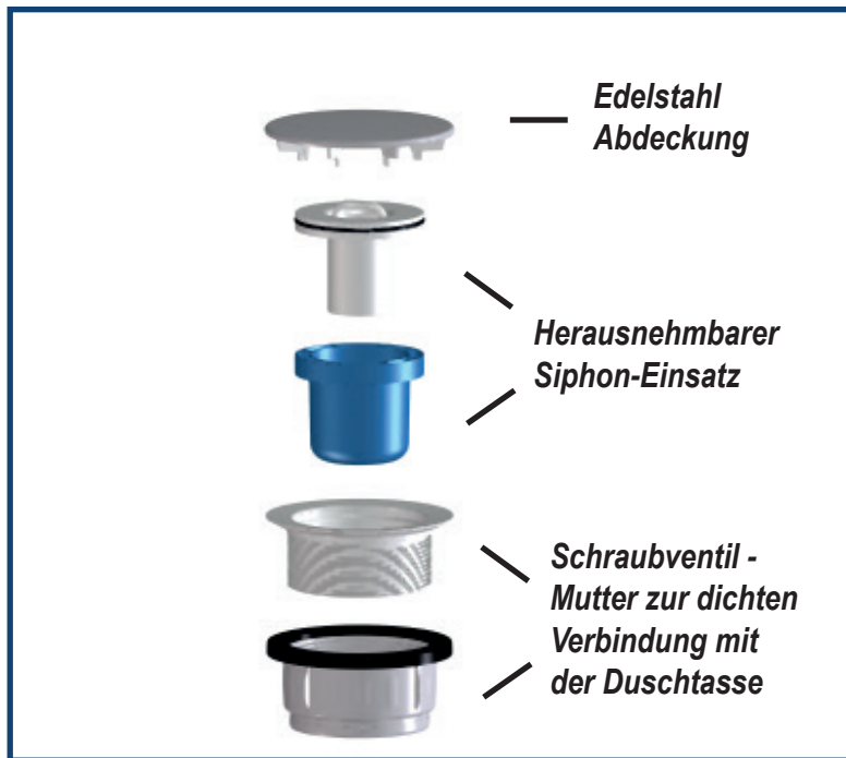
— Komplettier-Set
