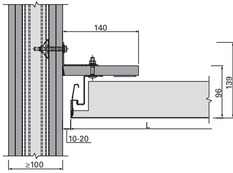
A-A | Anschluss an GK-Wand | flurlängsseitig | u138544
