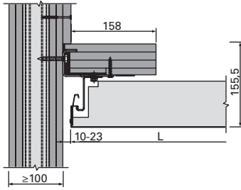
A-A | Anschluss an GK-Wand | flurlängsseitig | u144345
