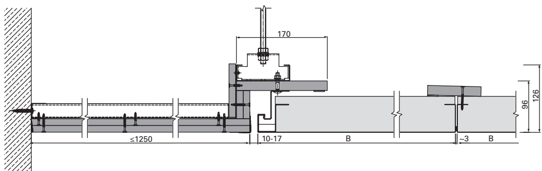
F-F | Anschluss an GK-Fries höhengleich | mit 3-seitiger Einhängekantung | flurstirnseitig | u137360
