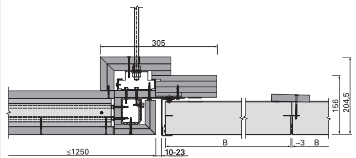
F-F | Anschluss an GK-Fries | flurstirnseitig | u147007
