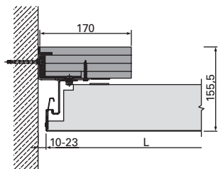
A-A | Anschluss an Beton-/Massivwand | flurlängsseitig | u146987
