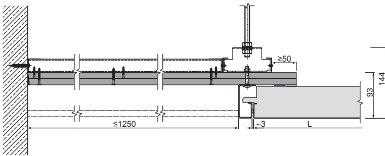
E-E | Anschluss an GK-Fries höherliegend | flurlängsseitig | u43064
