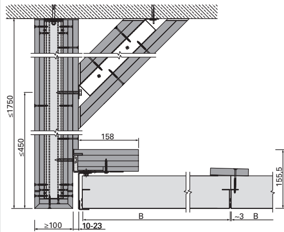
B-B | Anschluss an GK-Schürze | flurstirnseitig | u145049
