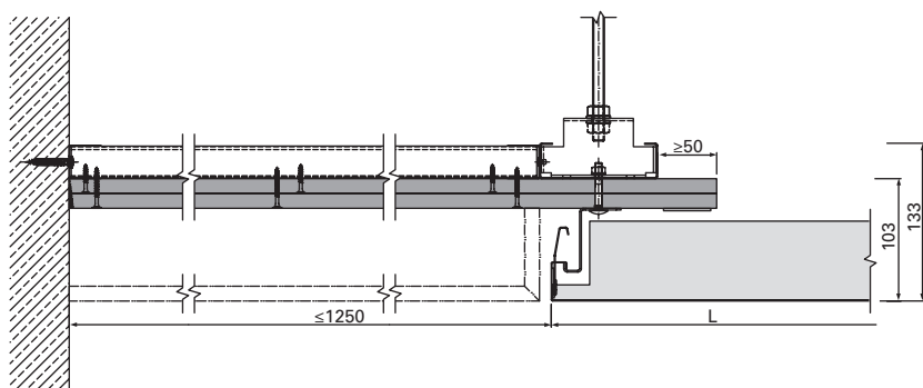
E-E | Anschluss an GK-Fries höherliegend | flurlängsseitig | u138561
