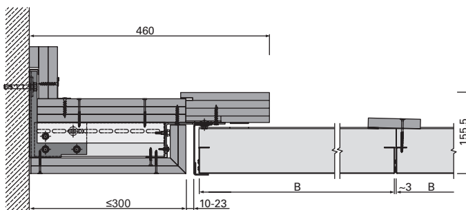
D-D | Anschluss an Beton-/Massivwand | mit Frieskonsole Lindner - Flex | flurstirnseitig | u146999
