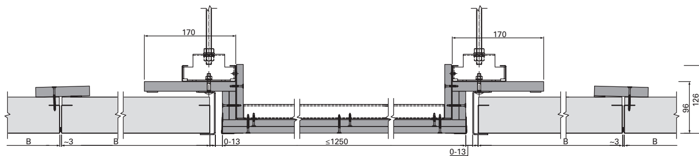
H-H | Flurerweiterung | GK-Mittelfries | flurstirnseitig | u137334
