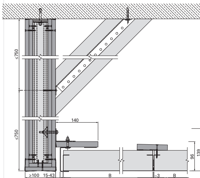
B-B | Anschluss an GK-Schürze | flurstirnseitig | u138556
