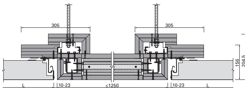
G-G | Flurerweiterung | GK-Mittelfries | flurlängsseitig | u147009
