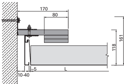
A-A | Anschluss an Beton-/Massivwand | flur-längsseitig | u43042
