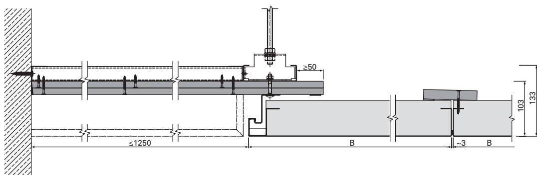
F-F | Anschluss an GK-Fries höherliegend | mit 3-seitiger Einhängekantung | flurstirnseitig | u137359
