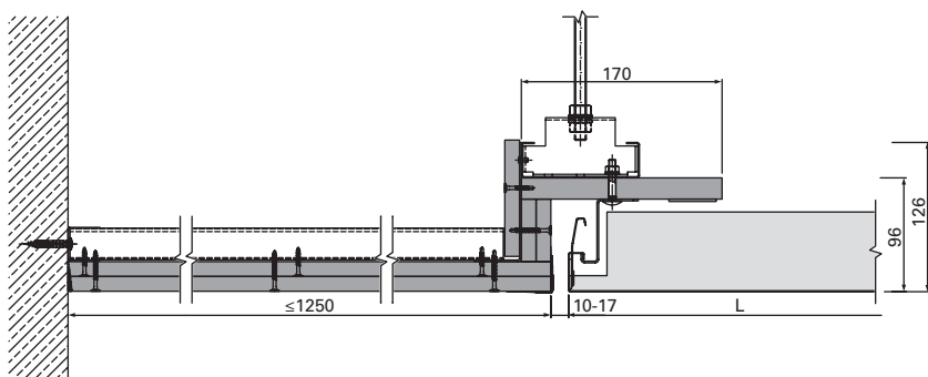
E-E | Anschluss an GK-Fries höhengleich | flurlängsseitig | u138563
