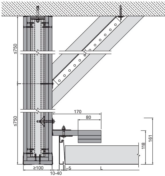
A-A | Anschluss an GK-Schürze | flurlängsseitig | u139175
