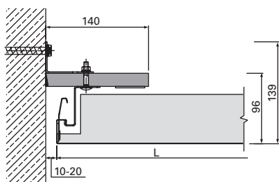
A-A | Anschluss an Beton-/Massivwand | flurlängsseitig | u138543
