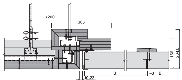
F-F | Anschluss an GK-Decke | flurstirnseitig | u147008
