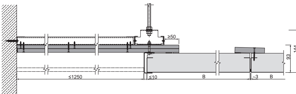
F-F | Anschluss an GK-Fries höherliegend | flurstirnseitig | u138605
