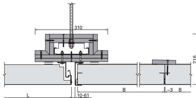
J-J | Flurerweiterung | Mittenabhängung | u147012
