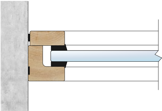
Wandanschluss Schnitt D-D
