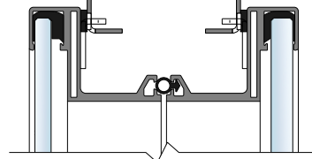
T-Stoß
