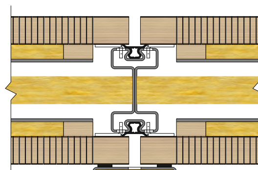
T-Stoß
