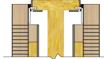
T-Stoß
