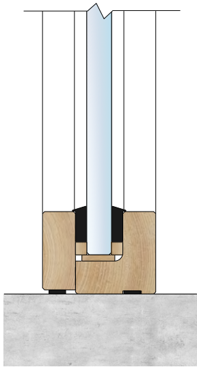
Bodenanschluss Schnitt C-C
