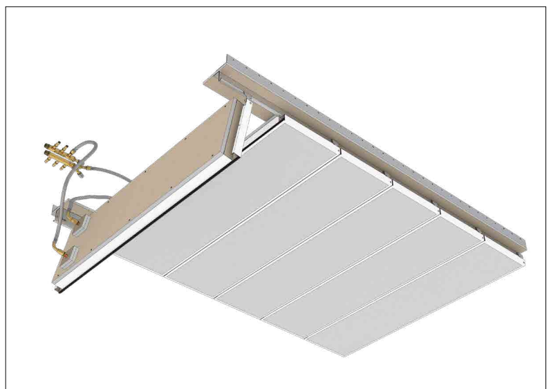
Ansicht von unten Plafotherm® F30-AB Typ 8.1
