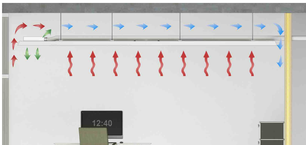
Funktionsweise Plafotherm® DS AirHybrid
