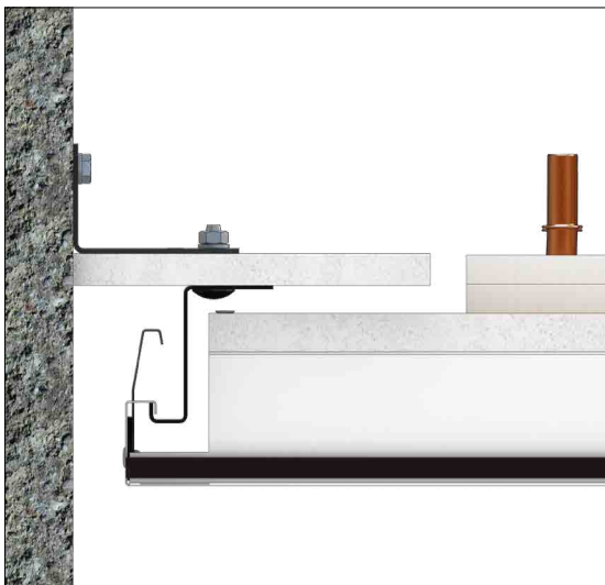
Schnit Plafotherm® F30-AB Typ 8.1
