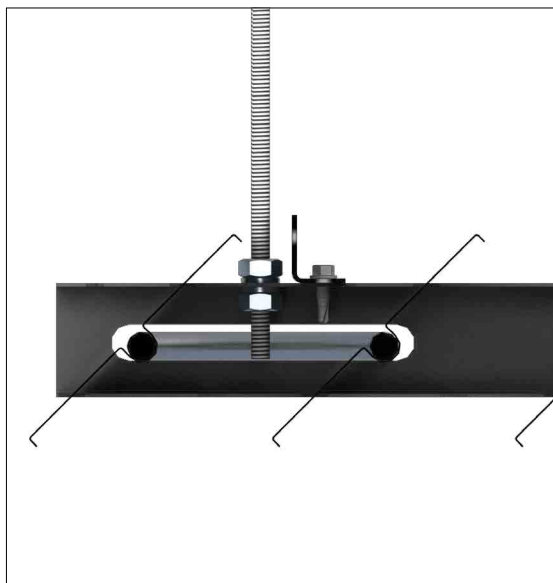
Schnitt Plafotherm® KN eco
