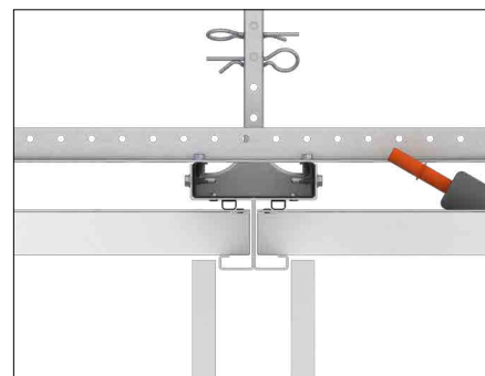
Schnitt Plafotherm® B 147 SD Typ 1
