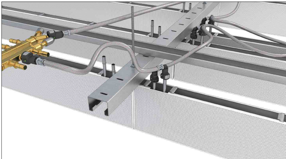
Detail Plafotherm® L 609 Typ 1
