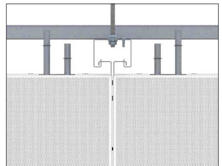
Schnitt Plafotherm® L 609 Typ 1
