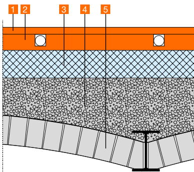
Niveausgleich auf Gewölbedecke mit fermacell® Therm25™ Element (Bauphysik ist zu beachten)
