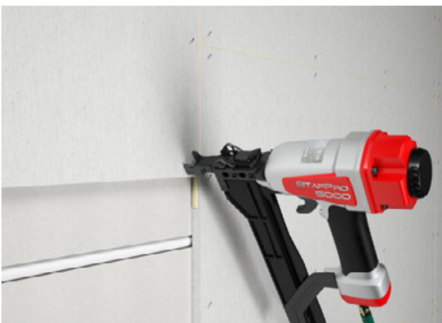
Befestigung zusätzliche Lage fermacell® Gipsfaserplatte oder Powerpanel H 2 O inkl. Fugenausbildung
