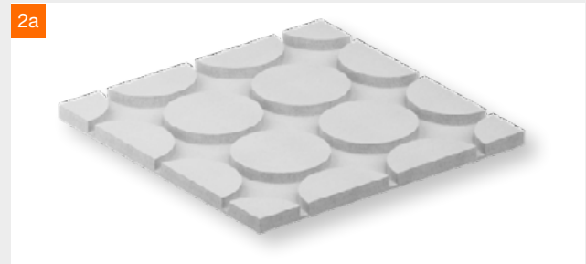
fermacell® Therm25™-167 Element rund, ergänzendes Element bei speziellen Grundrissen oder Türdurchgängen, Nutabstand 167 mm.
