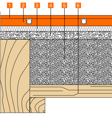
Niveausgleich der Holzbalkendecke mit tragfähigem Einschub mit fermacell® Therm25™ Element
