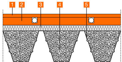
Stahltrapezdecke mit fermacell® Therm25™ Element
