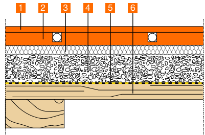
Niveausgleich auf Holzbalkendecke mit fermacell® Therm25™ Element
