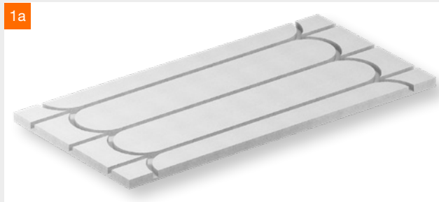
fermacell® Therm25™-167 Standard-Platte mit Fräsungen für die Längsverlegung mit Umlenk-Nuten, Nutabstand 167 mm.
