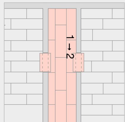
Verlegeschema Flurbereich (Details Türdurchgang siehe Kapitel 7.2)
