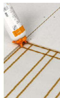
Kleberschnur am Rand der Platte
