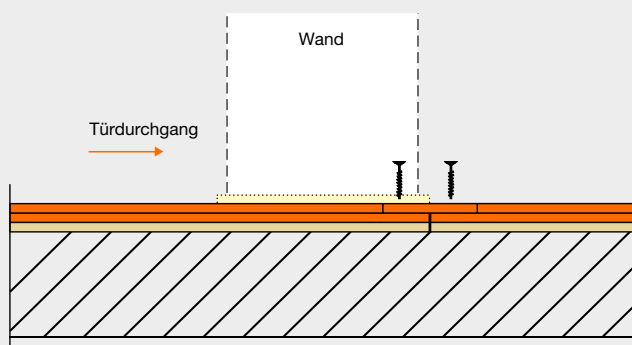
3. Streifen aus fermacell® Gipsfaserplatte und Estrichelement kraftschlüssig miteinander verbinden, z. B. mit fermacell™ Schnellbauschrauben oder Spreizklammern. Der Abstand der Verbindungsmittel darf max. 150 mm betragen
