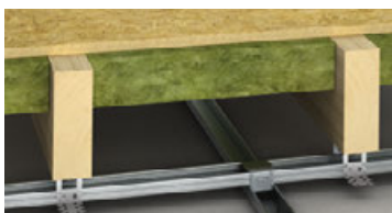
Geschlossene Holzbalkendecke, Unterdecke federnd abgehängt
