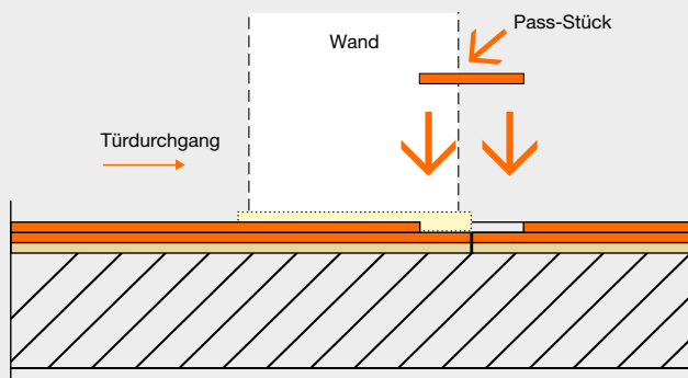
2. In geeigneter Länge, Breite und Dicke einen Streifen aus einer fermacell® Gipsfaserplatte ausschneiden. fermacell™ Estrichkleber auf den Falz auftragen und anschließend das Pass-Stück einsetzen
