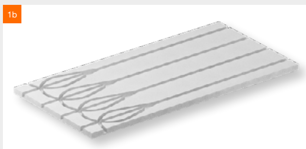
fermacell® Therm25-125™ Element, Fräsungen mit Umlenk-Nuten und geringerem Rohrabstand für eine verbesserte Wärmeleistung, z.B. für Badezimmer, Nutabstand 125 mm.
