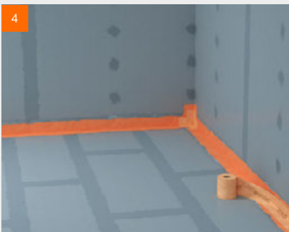
4 In die feuchte Flüssigfolie das fermacell™ Dichtband eindrücken
