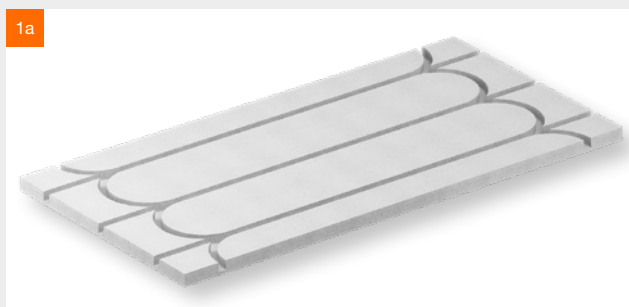
fermacell® Therm25™-167 Standard-Platte mit Fräsungen für die Längsverlegung mit Umlenk-Nuten, Nutabstand 167 mm.
