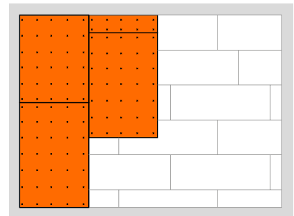
Befestigung der 3. Lage am Beispiel Gipsfaserplatte auf fermacell® Gipsfaser Estrichelementen
