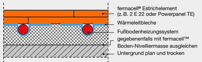
Beispiel 2: fermacell® Gipsfaser Estrichelement 2 E 22 oder fermacell® Powerpanel TE auf Warmwasser-Fußbodenheizung
