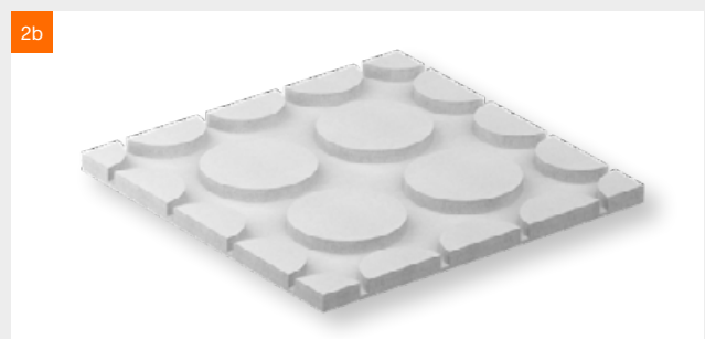
fermacell® Therm25-125™ Element rund, ergänzendes Element mit Fräsungen mit geringerem Rohrabstand für eine verbesserte Wärmeleistung, z.B. für Badezimmer, Nutabstand 125 mm.
