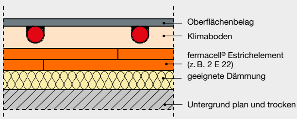
Beispiel 1: Klimaboden auf fermacell® Gipsfaser Estrichelement 2 E 22
