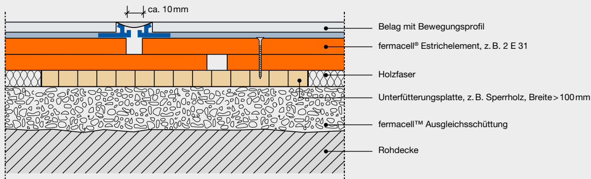
Bewegungsfuge auf fermacell™ Ausgleichsschüttung mit fermacell® Gipsfaser oder TE Estrichelement
