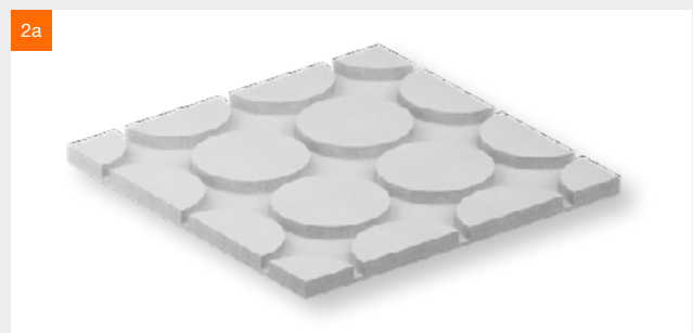
fermacell® Therm25™-167 Element rund, ergänzendes Element bei speziellen Grundrissen oder Türdurchgängen, Nutabstand 167 mm.
