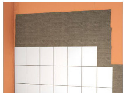
Abb. 9: Verfliesung mit fermacell™ Flexkleber im Dünnbettverfahren auf vollflächiger Abdichtung
