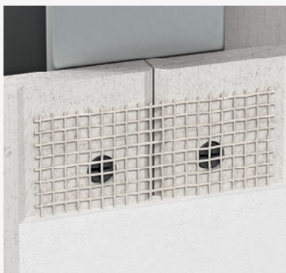
Trockenbau-Kante
