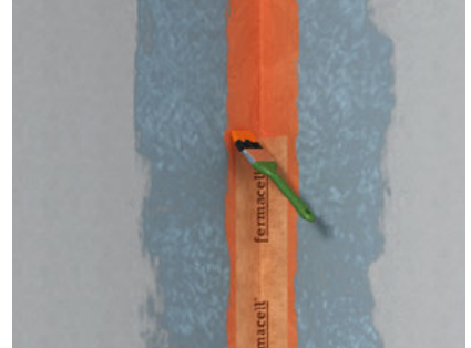
Abb. 2+3: fermacell™ Dichtband in die zuvor aufgetragene, noch feuchte fermacell™ Flüssigfolie drücken und direkt mit Flüssigfolie überstreichen – Trocknungszeit mind. 1 Stunde
