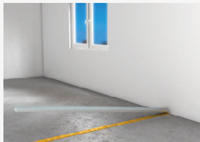
Auslegen der UW-Anschlussprofile am Boden auf Dämmstreifen
