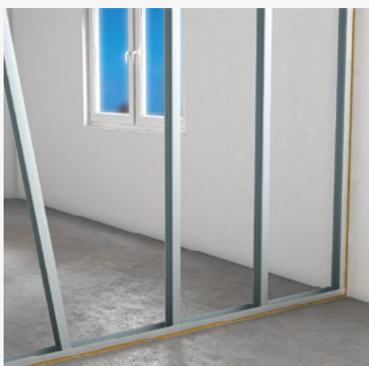
Montage der CW-Ständerprofile
