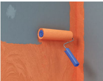
Abb. 7: Sicherstellung der Abdichtung für die Wassereinwirkungsklasse W1-I und W2-I. fermacell™ Flüssigfolie mit der Rolle mind. 2 x vollflächig auftragen (Trockenschichtdicke mindestens 0,5 mm). Gemäß DIN 18534-3 wird für den 2. Auftrag ein Farbunterschied zur besseren Nachvollziehbarkeit gefordert. 1. Auftrag: fermacell™ Flüssigfolie in Originalfarbe satt auftragen und trocknen lassen
