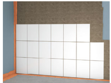
Abb. 6: Sicherstellung der Abdichtung für die Wassereinwirkungsklasse W0-I. Verfliesung mit fermacell™ Flexkleber im Dünnbettverfahren
