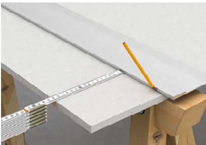
Einmessen
