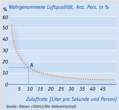
Abb. 2: Anteil Unzufriedener in Abhängigkeit von der Zulufrate
