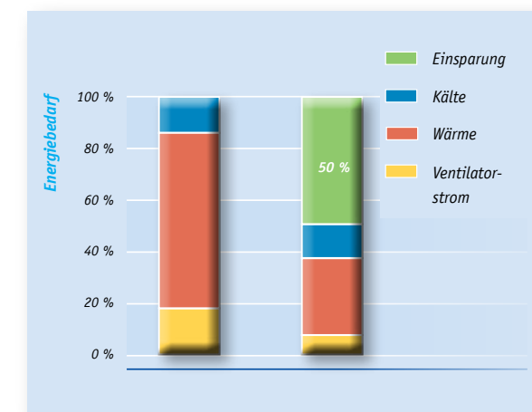
Energieeinsparung mit Bedarfslüftung
