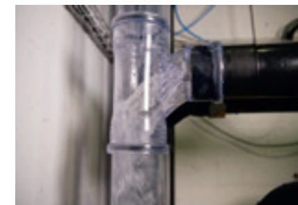
... und unter realen Bedingungen im Geberit Abwasserturm, der einen Teil des Prüflabors bildet, ist das identische Ergebnis sichtbar.
