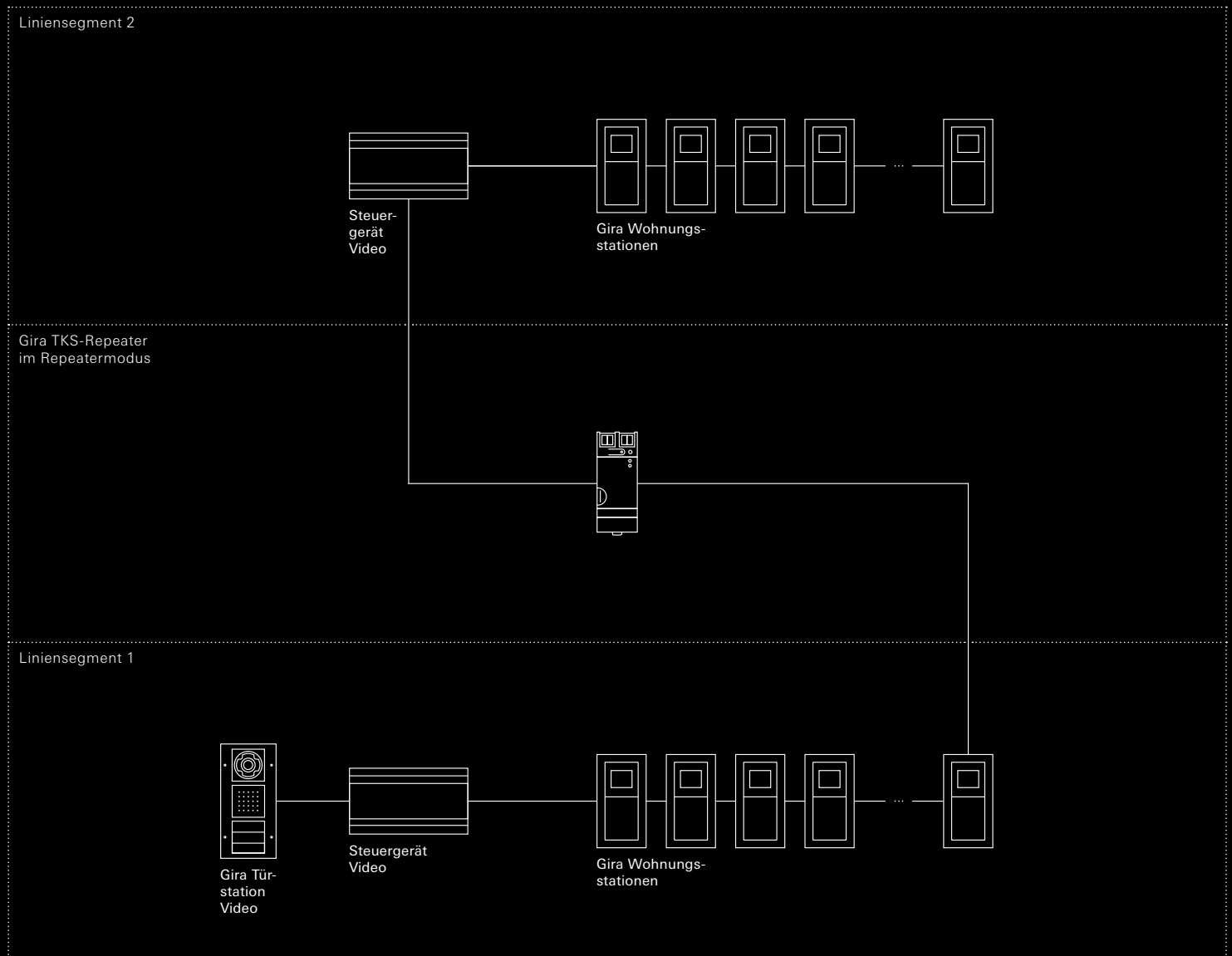
Systemübersicht TKS-Repeater
