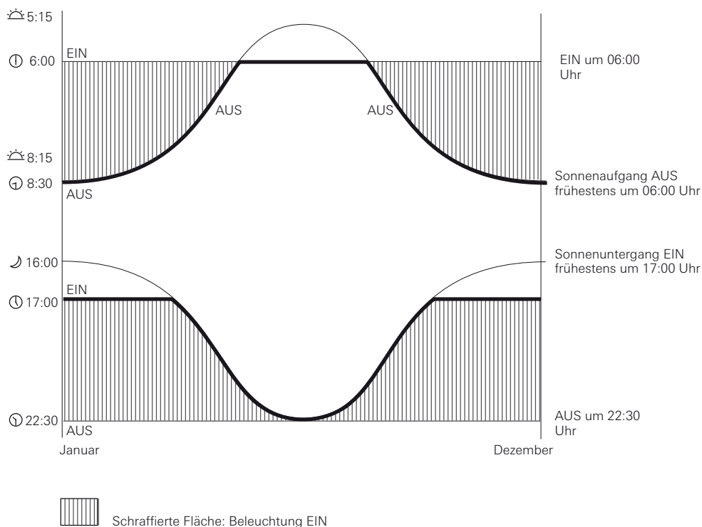
Bild 19 Verlauf der Astrofunktion
