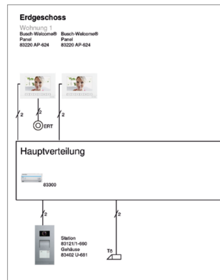
Übersichtsverbindungsplan
