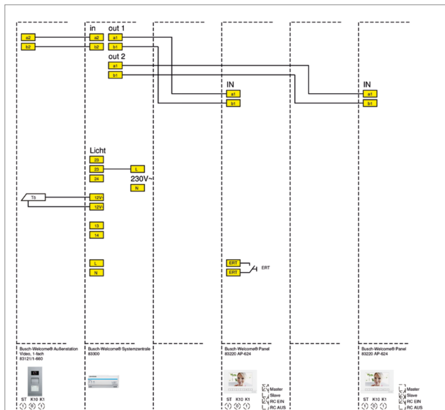
Außenschaltplan
