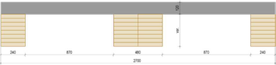
Querschnitt XC® office deck
