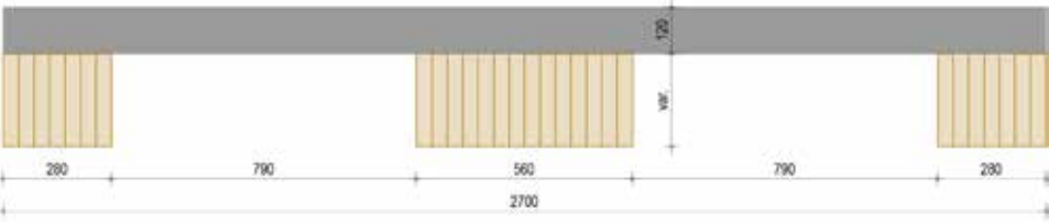
Querschnitt XC® office deck
