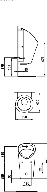
84019.2* Lema, siphonic urinal, concealed water inlet, with electronic control system, mains operated Lema, Absauge-Urinal, Zulauf innen, mit elektronischem Kontrollsystem, Netzbetrieb Lema, urinoir à effet siphonique, entrée d'eau intérieure, avec commande électronique, alimentation réseau Lema, orinatoio ad aspirazione, ingresso acqua nascosto, con sistema elettronico di controllo, alimentazione a rete
