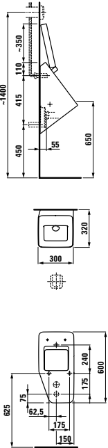
84090.5* Il Bagno Alessi dOt, siphonic urinal, with concealed water inlet, without cover Il Bagno Alessi dOt, Absauge-Urinal, Zulauf innen, Ausführung ohne Deckel Il Bagno Alessi dOt, urinoir à effet siphonique, entrée d'eau intérieure, version sans abattant Il Bagno Alessi dOt, orinatoio ad aspirazione, con ingresso acqua nascosto, modello senza coperchio
