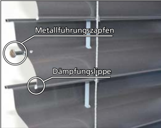
Lamellen werden wechselseitig durch vernietete Metallführungszapfen in den Schienen geführt
