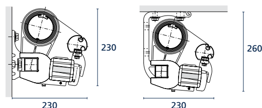
Wandmontage Deckenmontage
