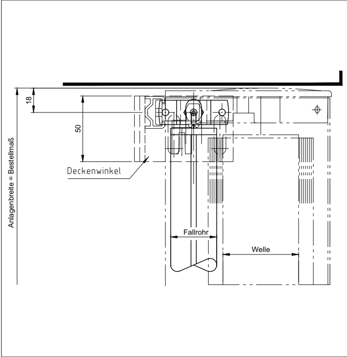
HORIZONTALSCHNITT DECKENMONTAGE
