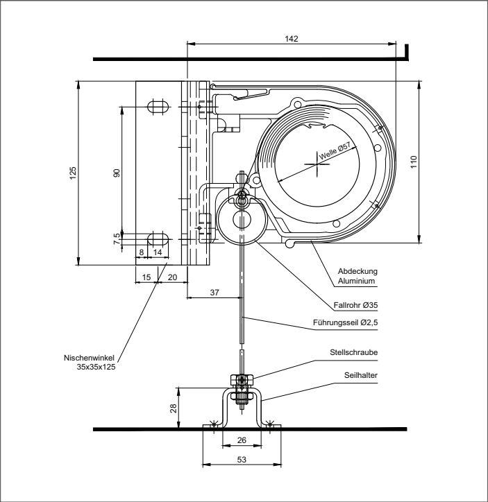
VERTIKALSCHNITT NISCHENMONTAGE
