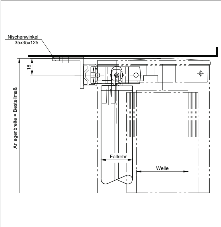
HORIZONTALSCHNITT NISCHENMONTAGE
