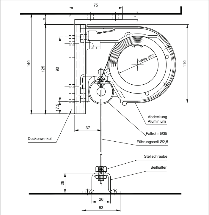
VERTIKALSCHNITT DECKENMONTAGE
