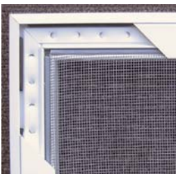
Eckverbinder (Außenansicht ohne Abdeckblende)
