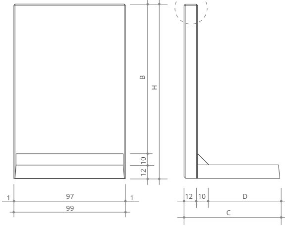
TYP 2 Höhen 130 - 155 cm
