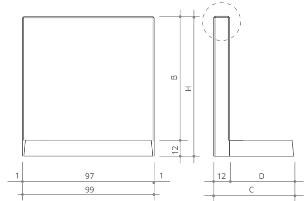
TYP 1 Höhen 55 - 105cm
