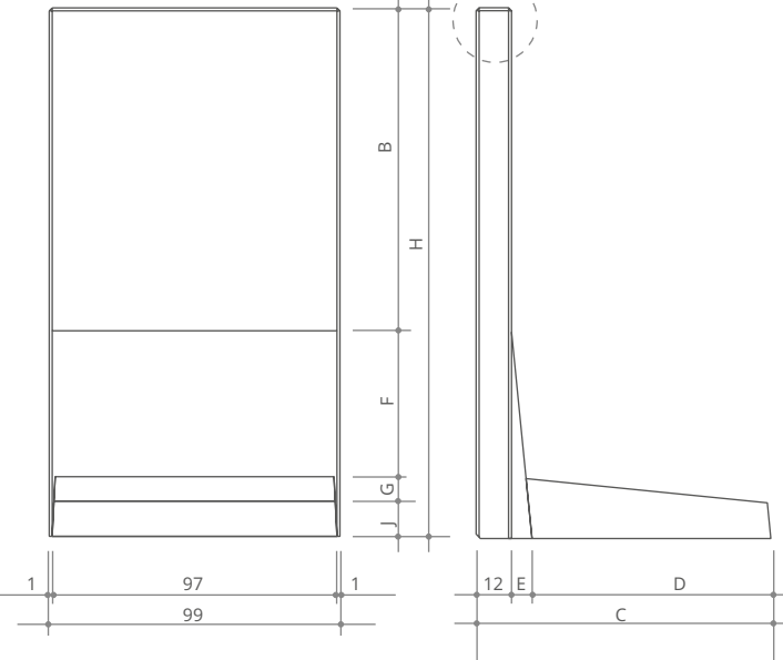
TYP 3 Höhen 180 - 405 cm
