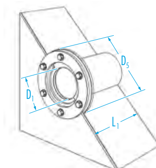
Variante: Curaflex® 4005/U als Sohlendurchführung
