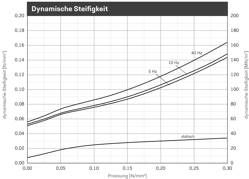
Verlauf der dynamischen Steifigkeit bei sinusförmiger Anregung um eine konstante Mittellast, Wegamplitude ± 0,25 mm. Probenabmessung 300 mm x 300 mm x 45 mm; Statische Steifigkeit als Tangentenmodul aus der Federkennlinie. Messung in Anlehnung an DIN 53513.
