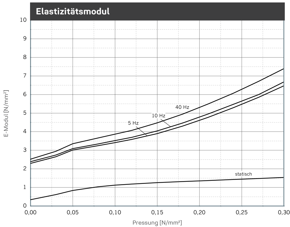
Verlauf des dynamischen E-Moduls bei sinusförmiger Anregung um eine konstante Mittellast, Wegamplitude ± 0,25 mm. Probenabmessung 300 mm x 300 mm x 45 mm; Statischer E-Modul als Tangentenmodul aus der Federkennlinie. Messung in Anlehnung an DIN 53513.
