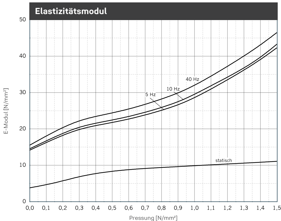
Verlauf des dynamischen E-Moduls bei sinusförmiger Anregung um eine konstante Mittellast, Wegamplitude ± 0,25 mm. Probenabmessung 200 mm x 200 mm x 40 mm; Statischer E-Modul als Tangentenmodul aus der Federkennlinie. Messung in Anlehnung an DIN 53513.
