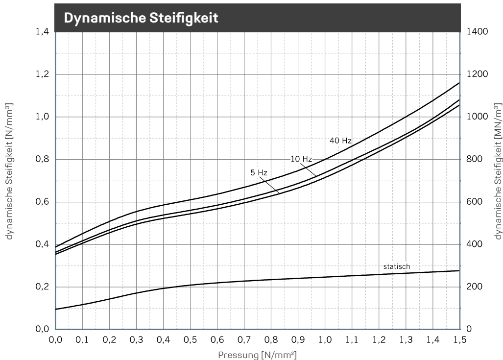
Verlauf der dynamischen Steifigkeit bei sinusförmiger Anregung um eine konstante Mittellast, Wegamplitude ± 0,25 mm. Probenabmessung 200 mm x 200 mm x 40 mm; Statische Steifigkeit als Tangentenmodul aus der Federkennlinie. Messung in Anlehnung an DIN 53513.
