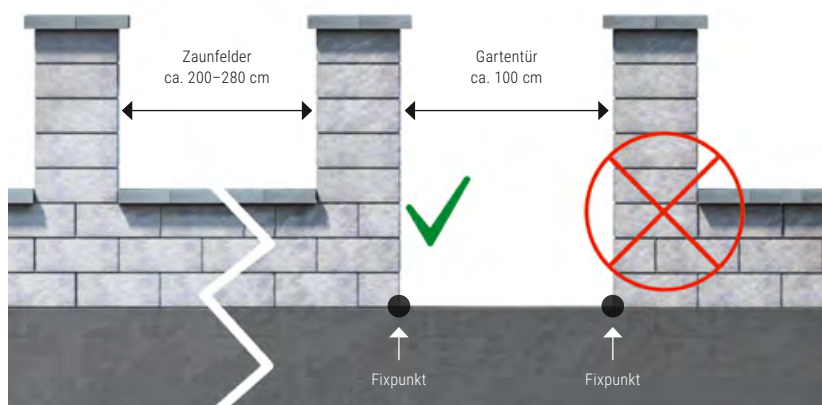
Abbildung 7: Planung
