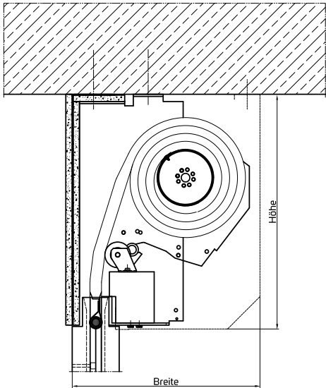
Deckenmontage V2
