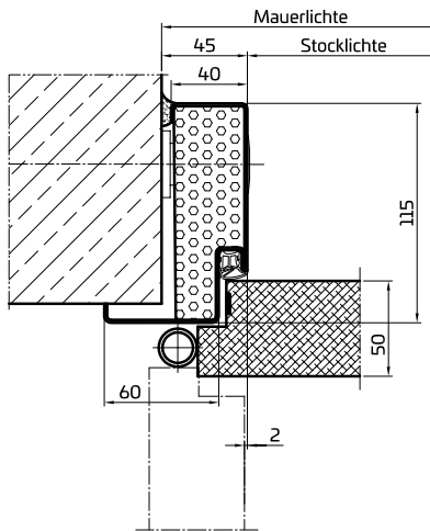
Beispiel: Betonwand
