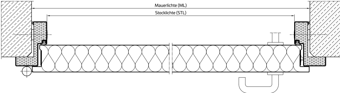
Drehflügeltor 1-flg. mit Eckzarge
