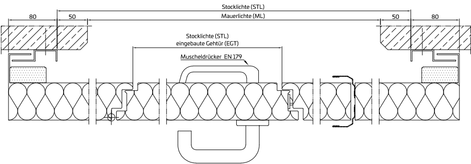
Schnelllaufftor 2-flg. mit eingebauter Gehrür, Betonwand
