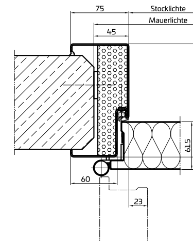
Beispiel: Betonwand
