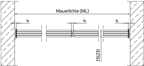
Horizontalschnitt
