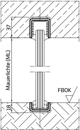
Vertikalschnitt
