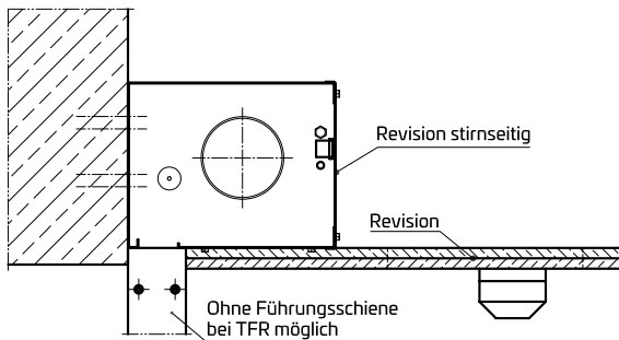
Gehäuse in der abgehängten Decke nicht sichtbar
