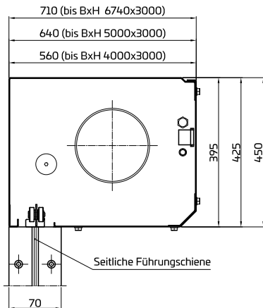
Maße TFF-EI V1
