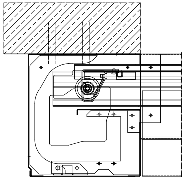
Einlaufprofil
