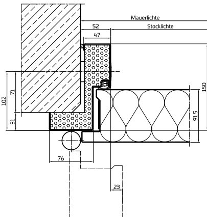
Beispiel: Betonwand
