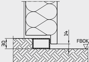
Aufbauschwelle FR 50 × 30 + Türblatt vierseitig
