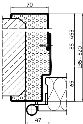
Umfassungszarge geteilt 00/30
