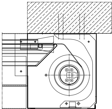
Wickelprofil
