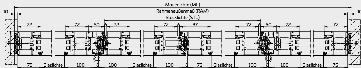
2-flügelig inkl. Seitenteile
