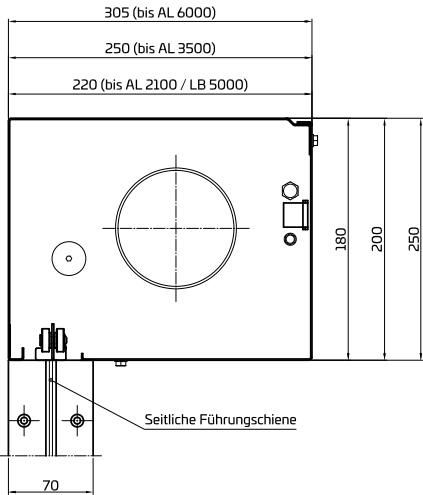
Maße TFF-EW
