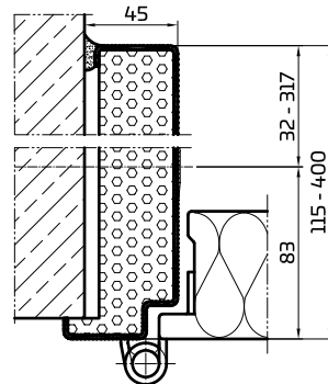
Umfassungszarge 00/30
