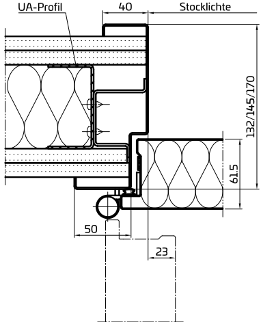
Beispiel: Trockenbauwand
