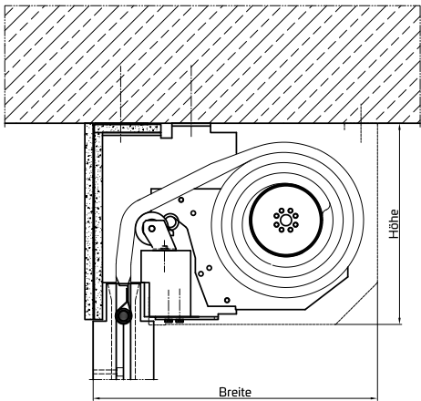
Deckenmontage V1
