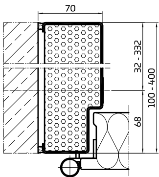
Umfassungszarge spiegelgleich 00/30
