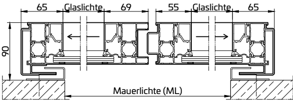
Horizontalschnitt 2-flügelig
