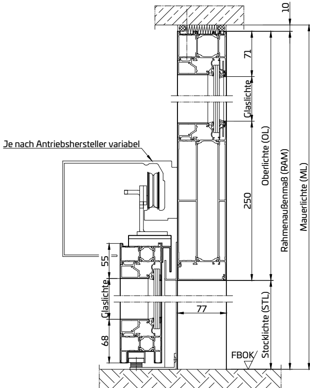
Vertikalschnitt mit Oberlichte
