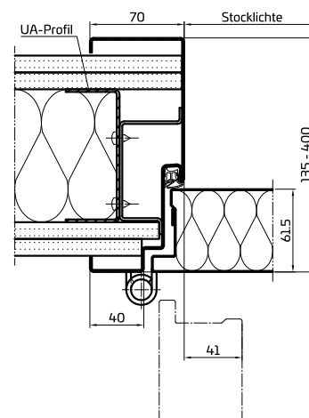
Beispiel: Trockenbauwand
