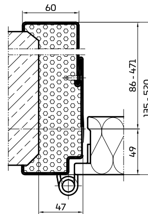
Umfassungszarge geteilt 00/30
