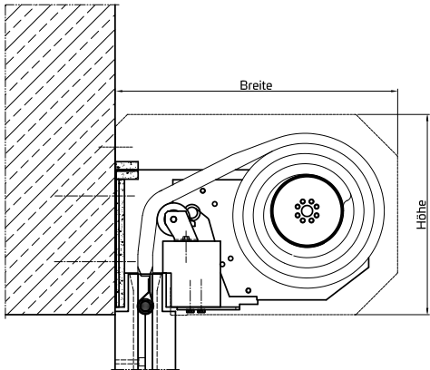
Deckenmontage V1
