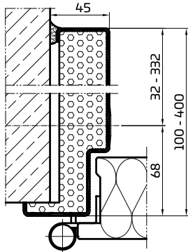
Umfassungszarge 00/30
