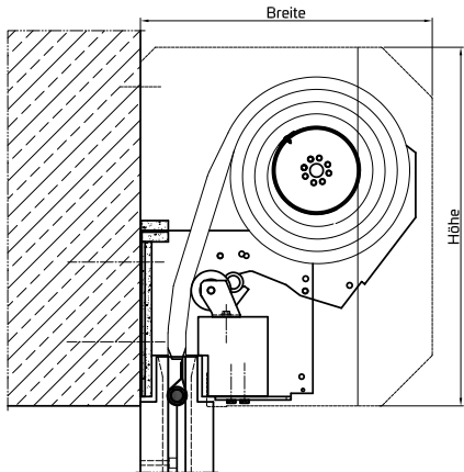
Wandmontage V2
