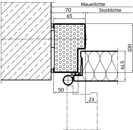
Beispiel: Betonwand mit Dübelmontage
