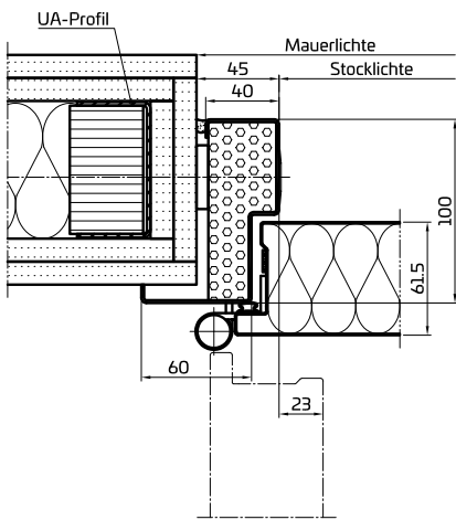
Beispiel: Trockenbauwand
