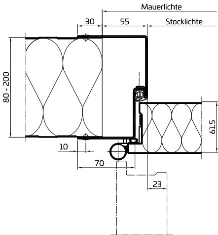
Beispiel: Paneelwand
