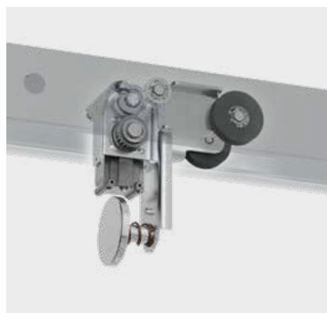
Freilauf Schiebetor
