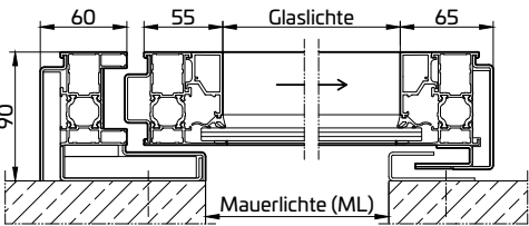
Horizontalschnitt 1-flügelig
