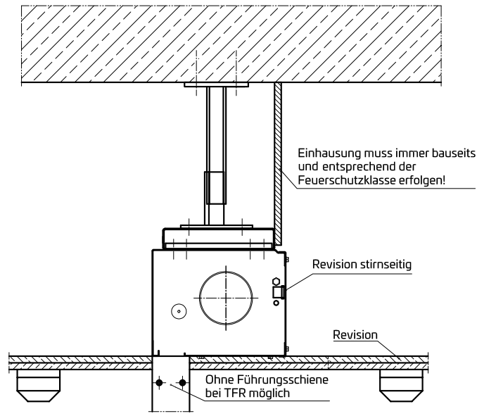
Gehäuse in der abgehängten Decke nicht sichtbar
