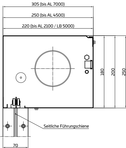
Maße TFF-E/TFR
