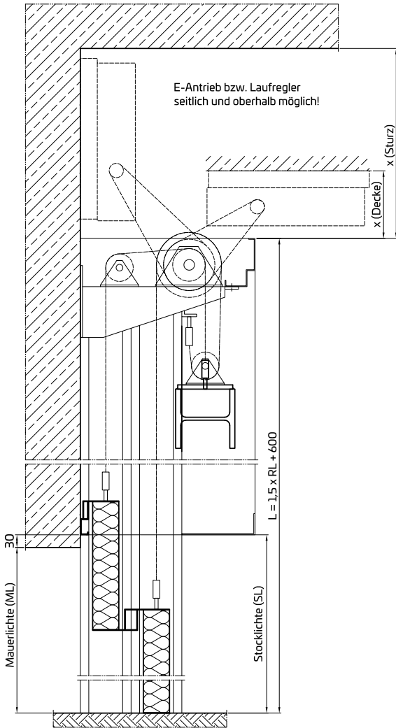
Teleskophubtor
