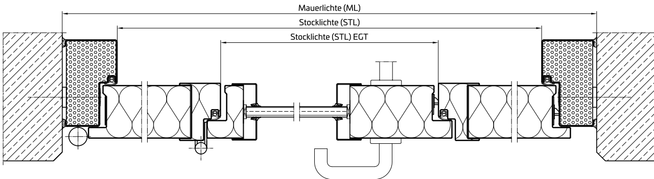
Drehflügeltor 1-flg. mit eingebauter Gehtür und Glasausschnitt
