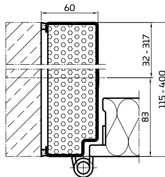
Umfassungszarge spiegelgleich 00/30
