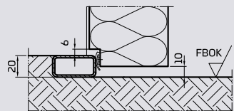
Bodendetail Außentür
