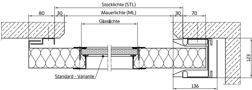
Schnelllaufftor 1-flg. mit Verglasung, Betonwand
