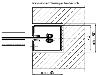
Seitliche Führung Nischenmontage
