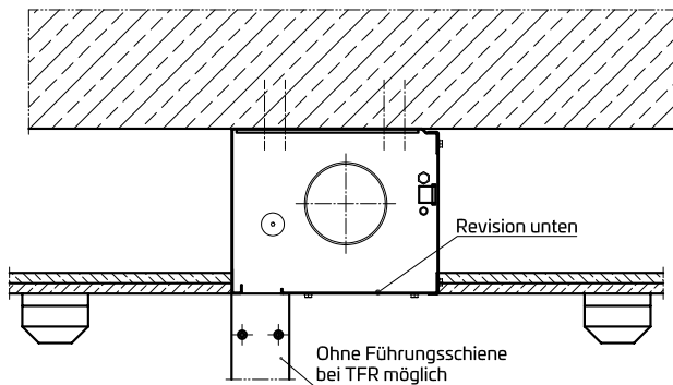
Gehäuse von unten sichtbar
