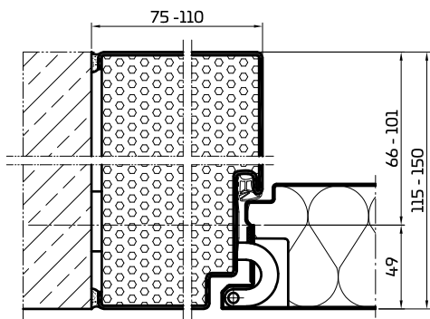
Blockzarge Variabel Betonwand mit Tectusband
