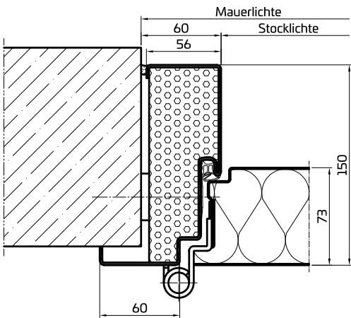
Beispiel: Wandbegleitender Einbau in Trockenbauwand
