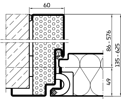
Umfassungszarge Leibungstief Betonwand mit Tectusband
