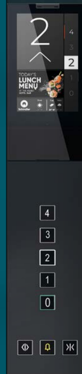
Kabinentableau, halbhoch, bündig, mit Kanalabdeckung aus obsidianschwarzem Laminat. Kanalabdeckung ist um ca. 5 mm zurückversetzt.
