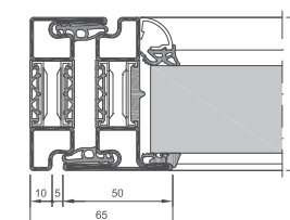
Türflügel-Blendrahmen
