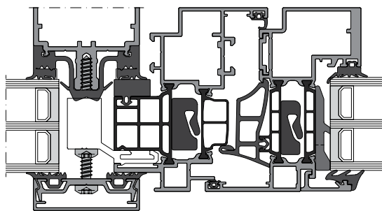
FRAME + 75 WA
