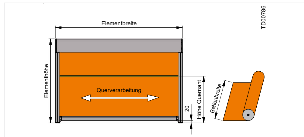
Querverarbeitung mit/ohne Naht je nach Elementhöhe (Elementbreite > ca. -Ballenbreite)
