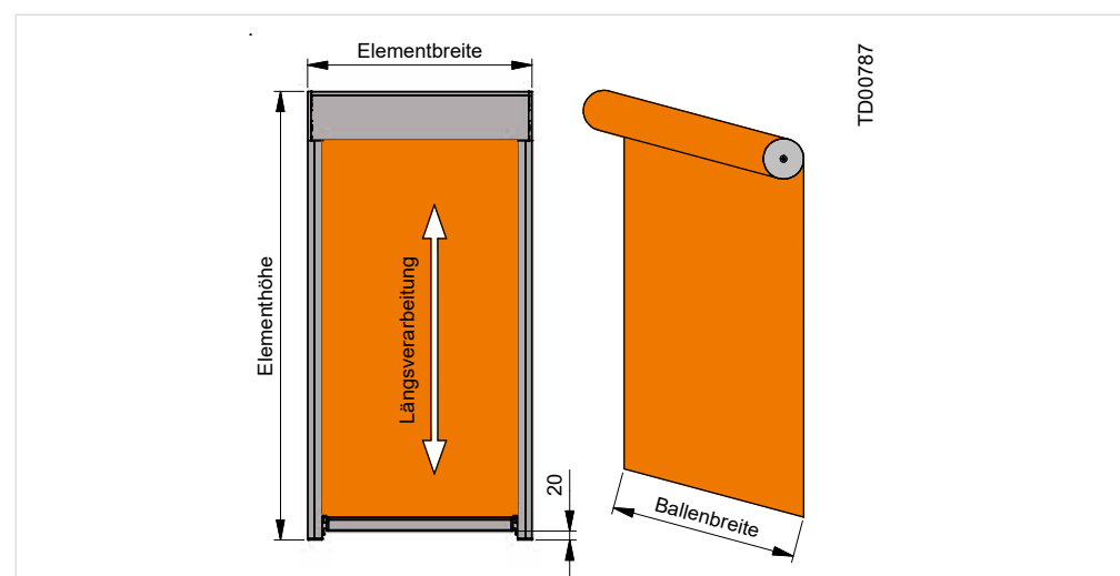
Längsverarbeitung ohne Naht (Elementbreite < ca. Ballenbreite)
